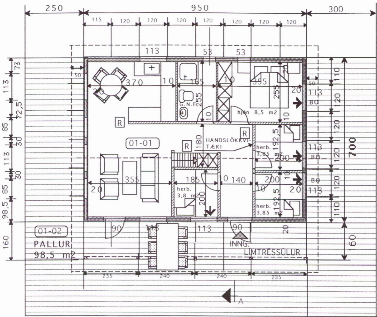
GRUNNMYND 1: 100
