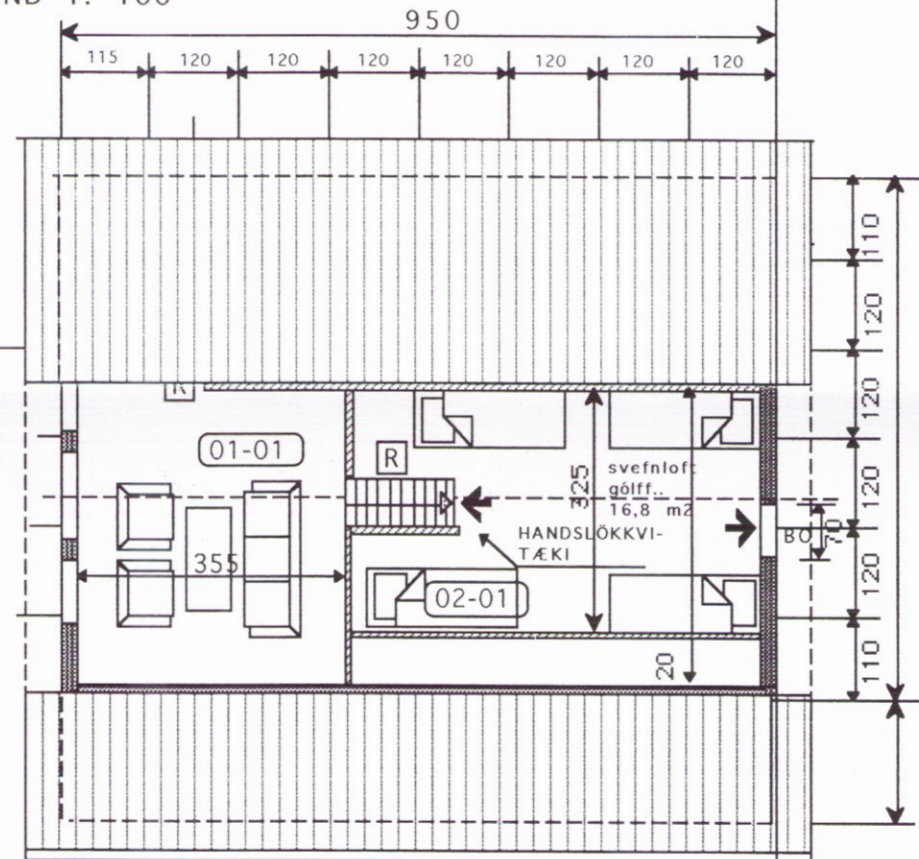
GRUNNMYND SVEFNLOFT 1: 100
