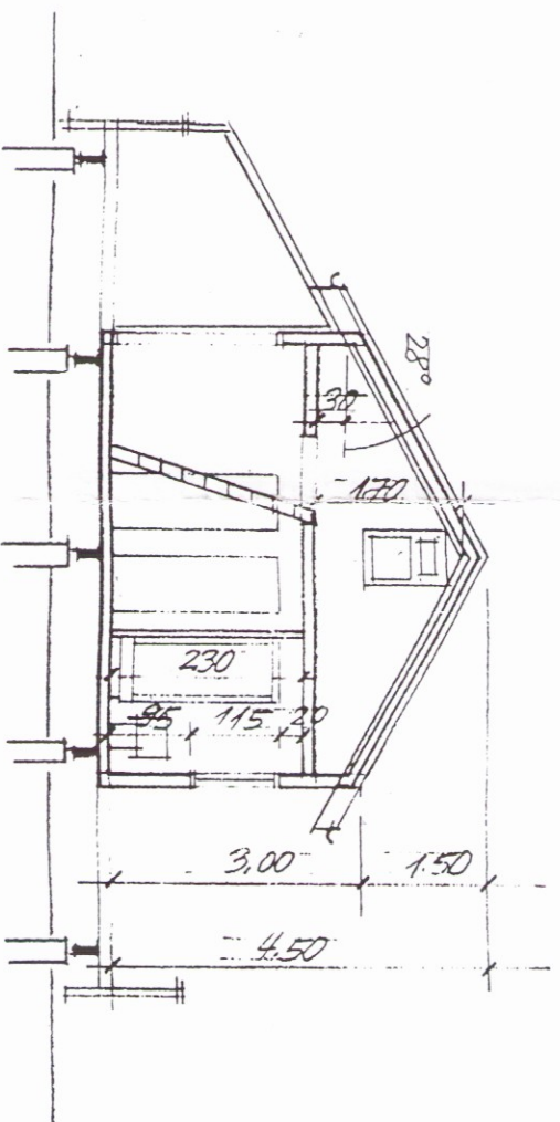
SKURÐUR A-A
