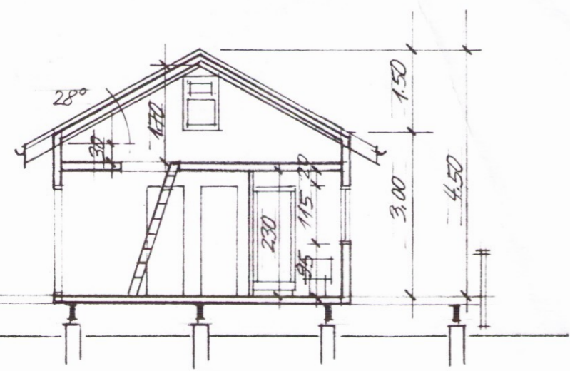
SKURÐUR A-A
