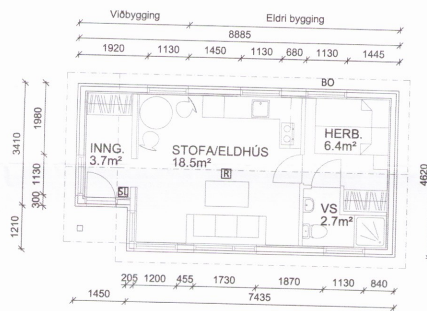
GRUNNMYND
