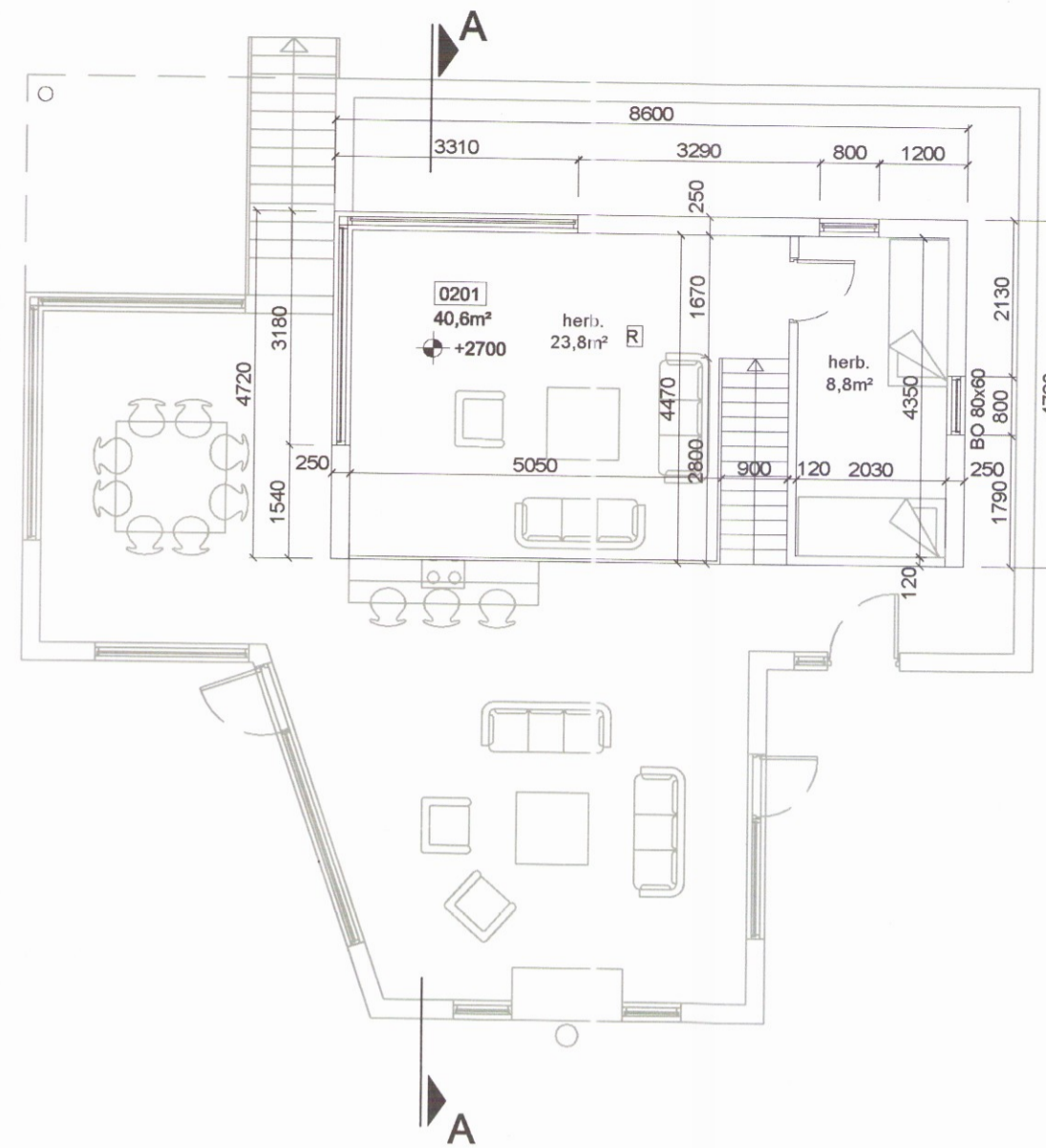
GRUNNMYND 2.HÆÐ 1:100
