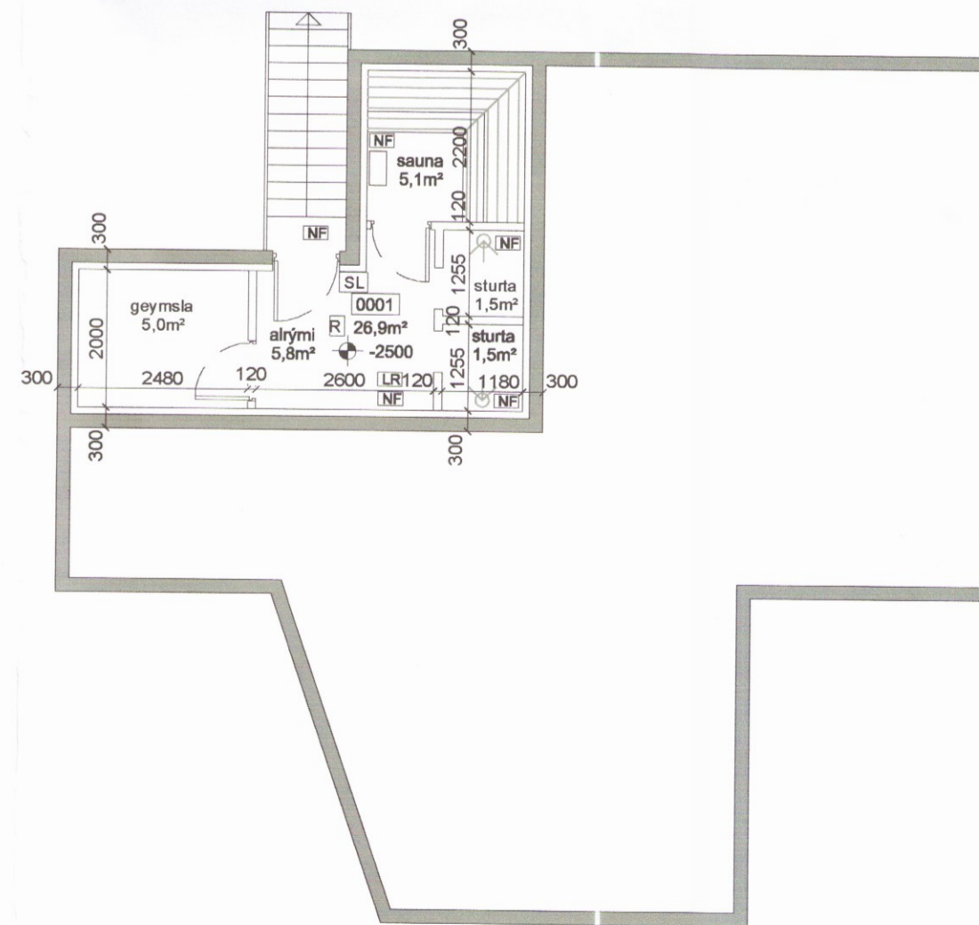
GRUNNMYND KJALLARI (SÖKKULL) 1:100
