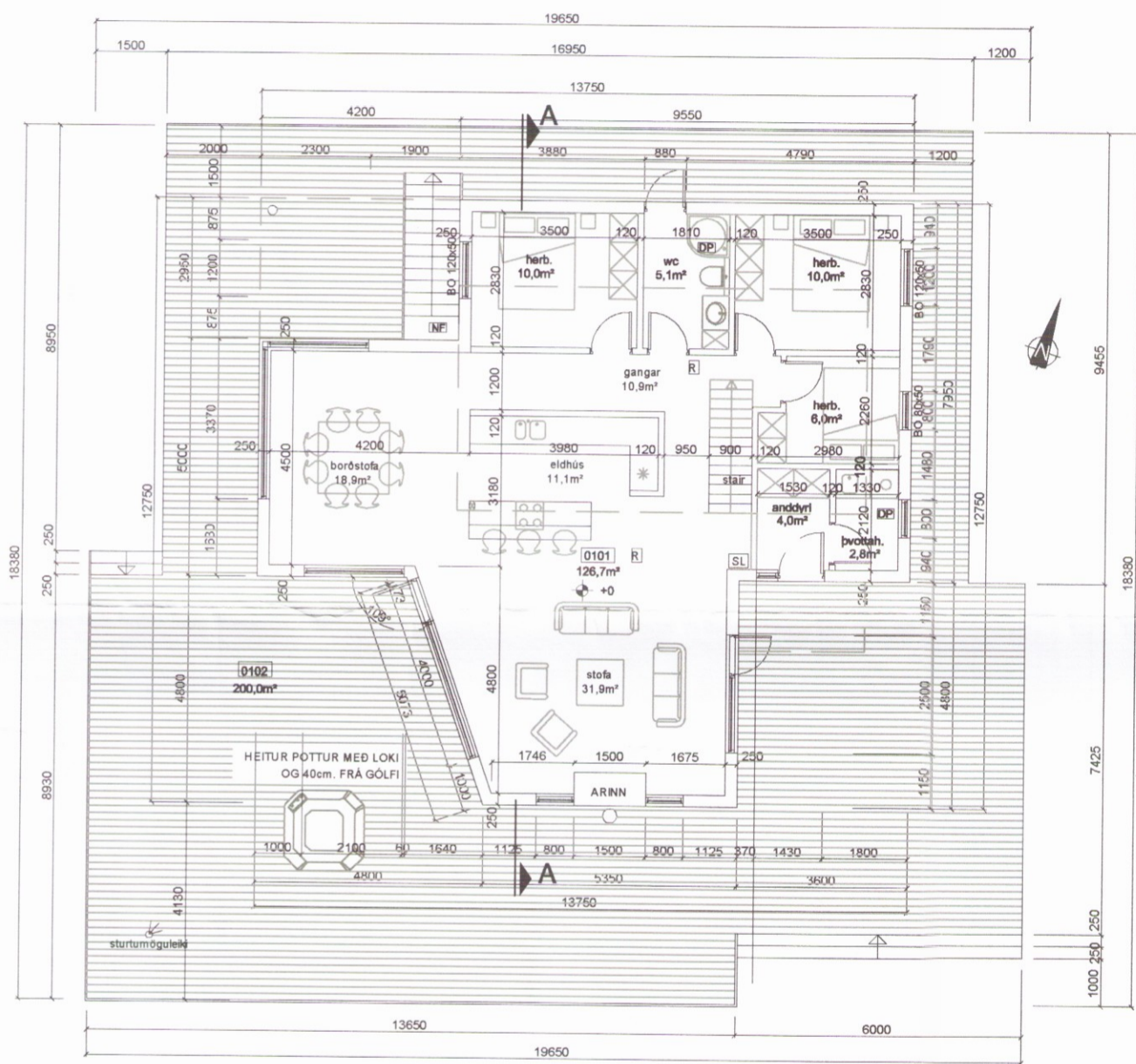
GRUNNMYND 1.HÆÐ 1:100
