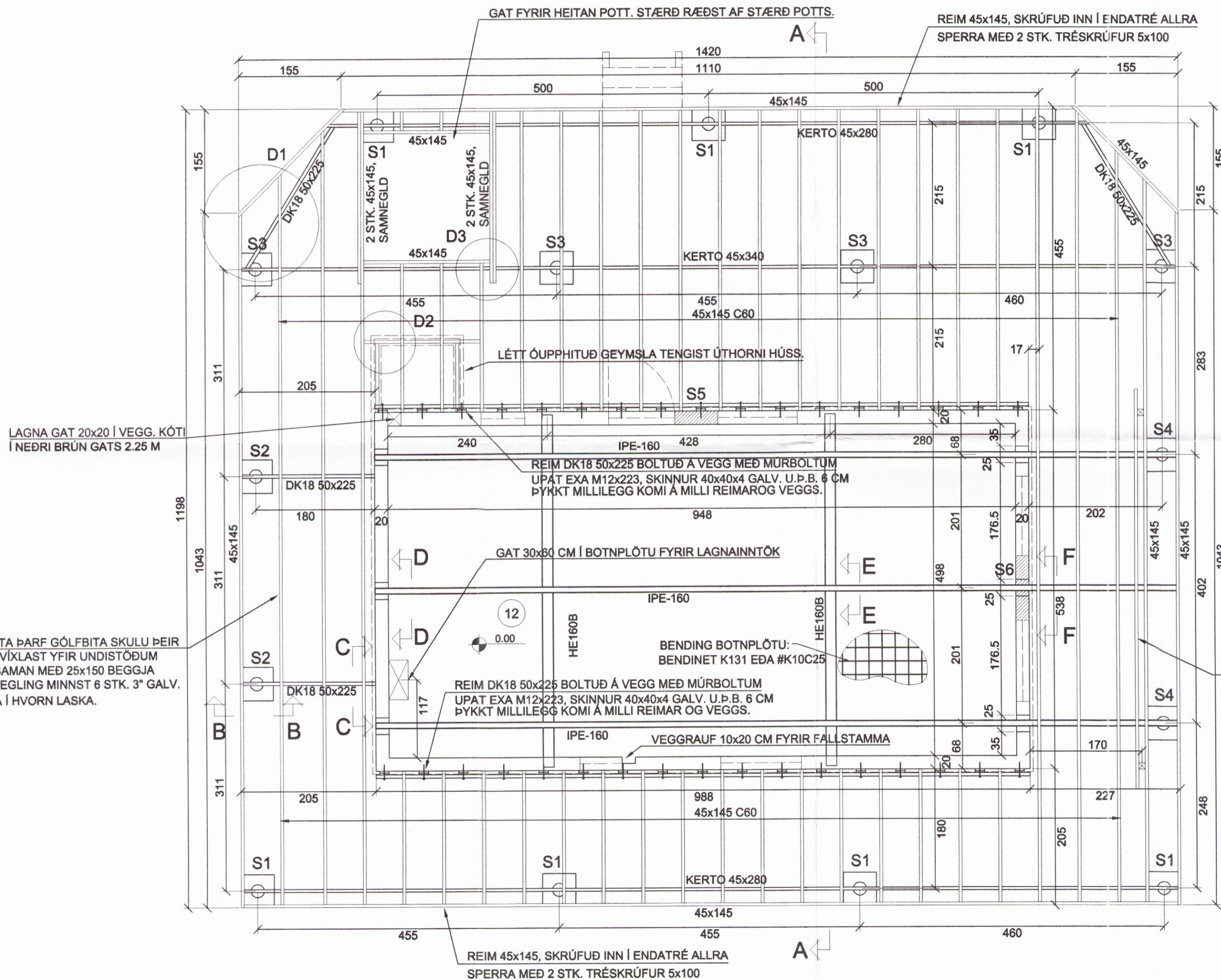
GRUNNMYND 1:50
