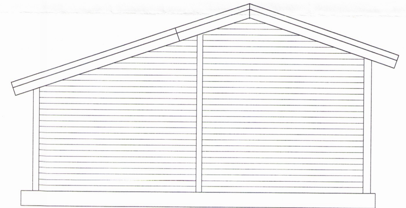
ÚTLIT NORÐVESTUR 1:50
