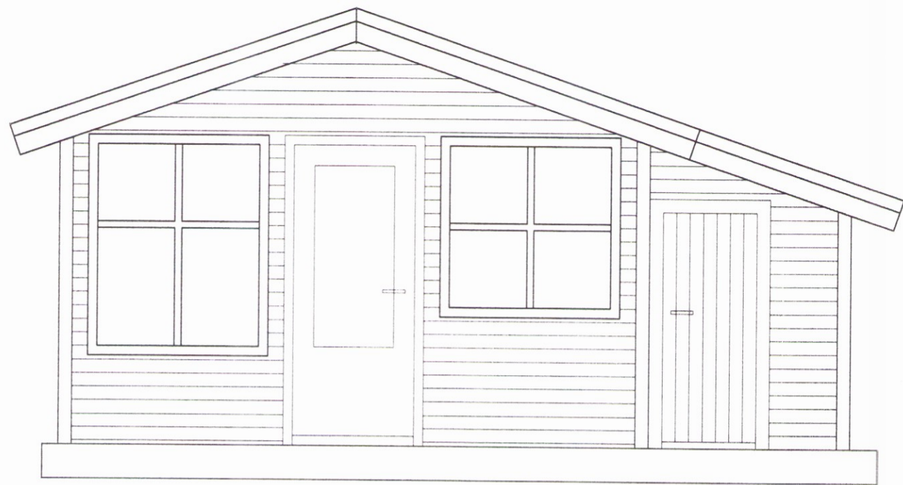
ÚTLIT SUÐVESTUR 1:50
