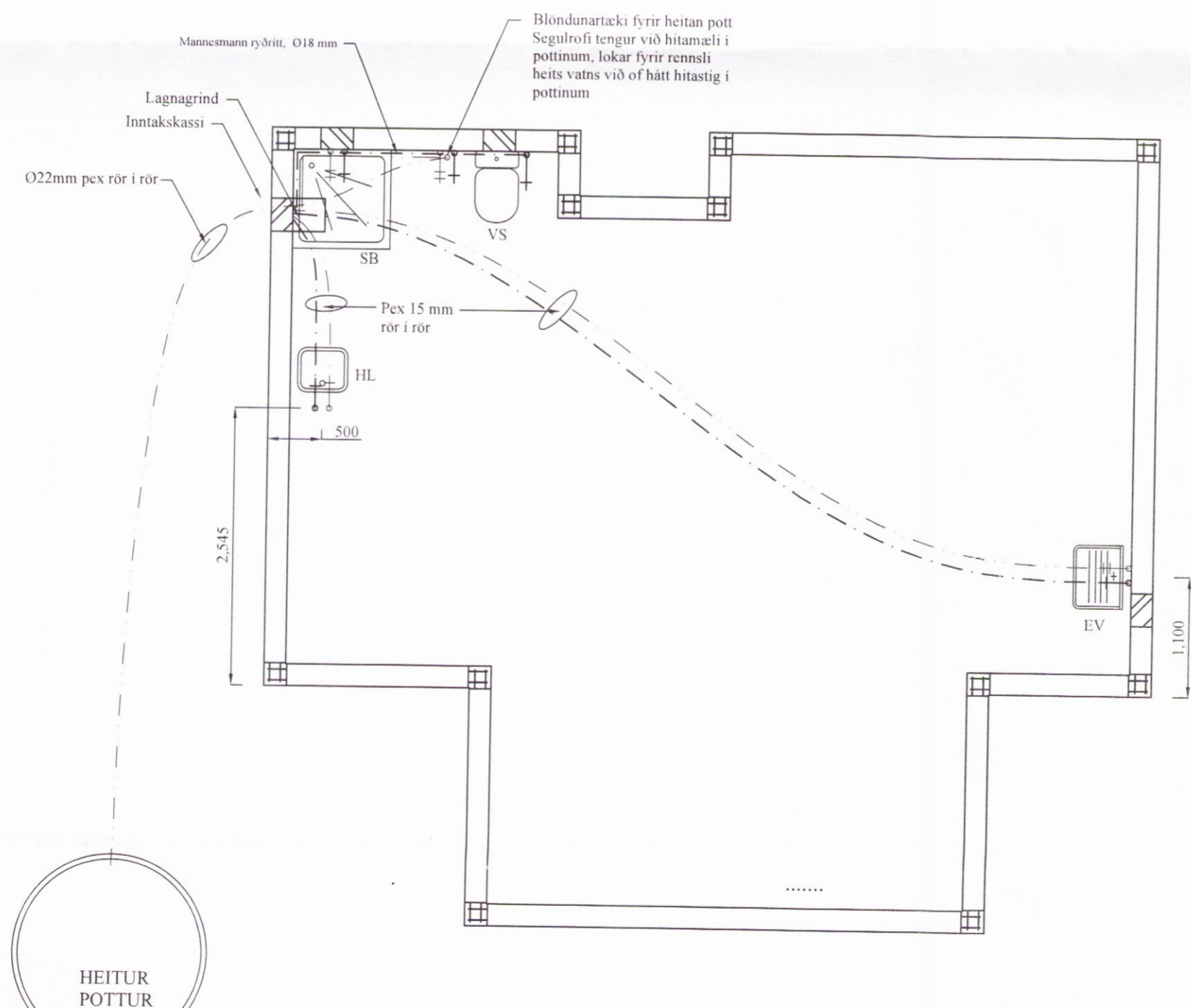
GRUNNMYND VATNSLAGNA Mkv. 1:50
