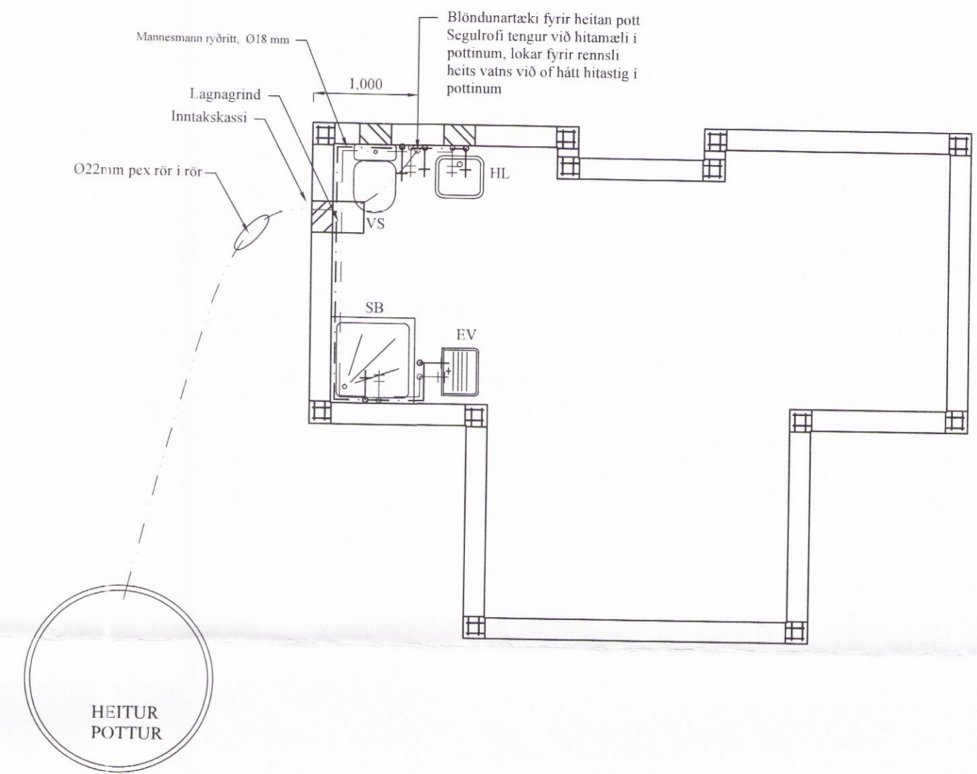
GRUNNMYND VATNSLAGNA Mkv. 1:50
