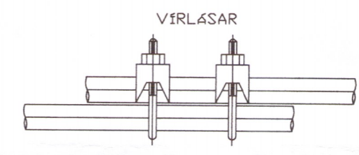
VÍRLÁSAR SAMTENGING STEYPUSTEINA SETJA SKAL TVÖ VÍRLÁSAR Á HVER SAMSEYTI
