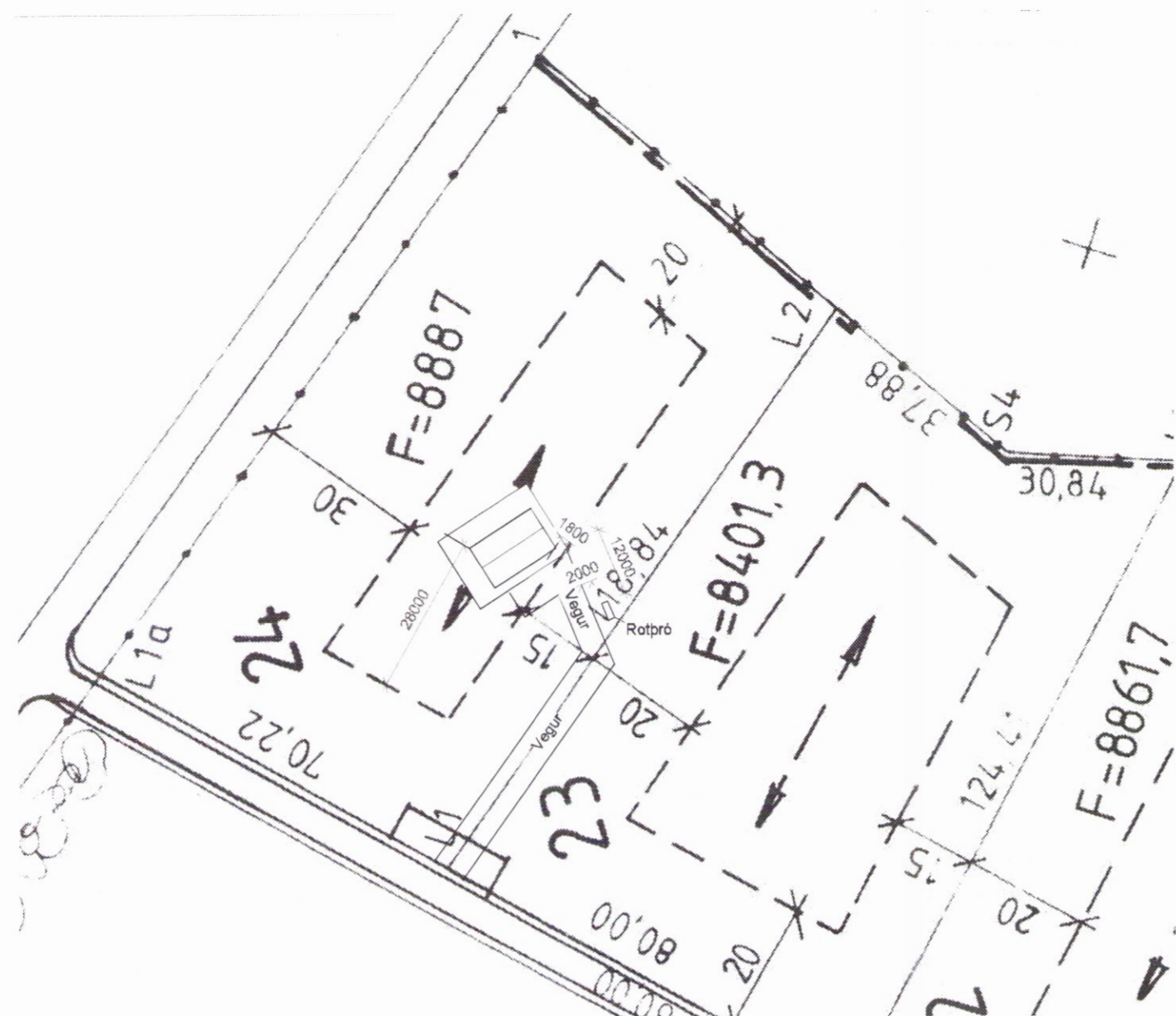
1 Afstöðumynd 1 : 1000
