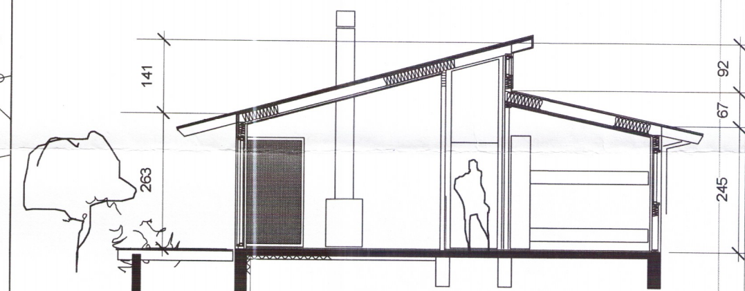
Sneiðing
