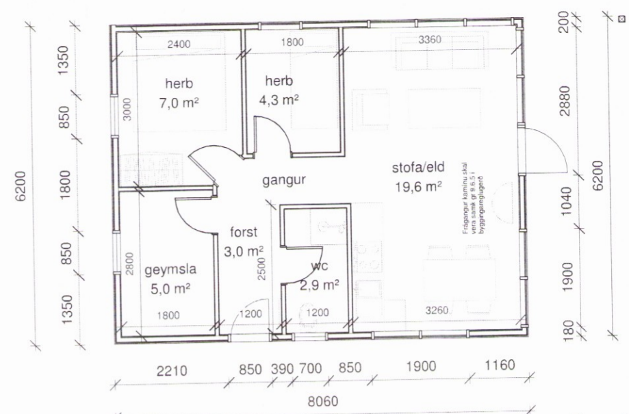
Grunnmynd núverandi 1 : 100
