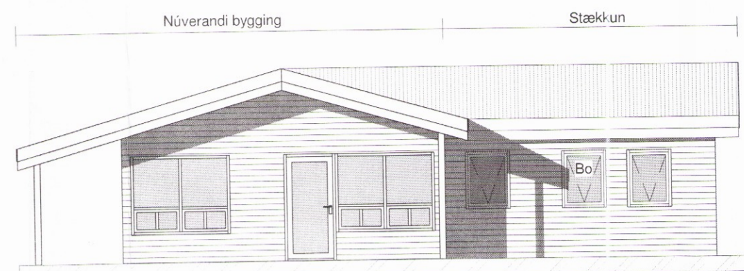
Austur 1 : 100
