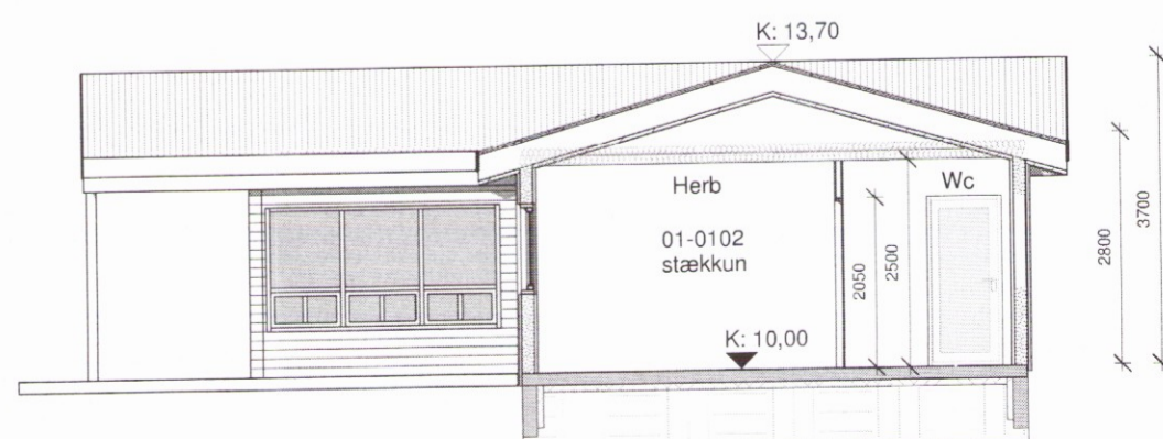
Snið A-A 1 : 100
