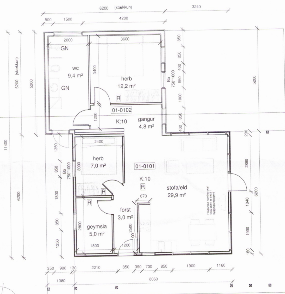
Grunnmynd með stækkun 1 : 100
