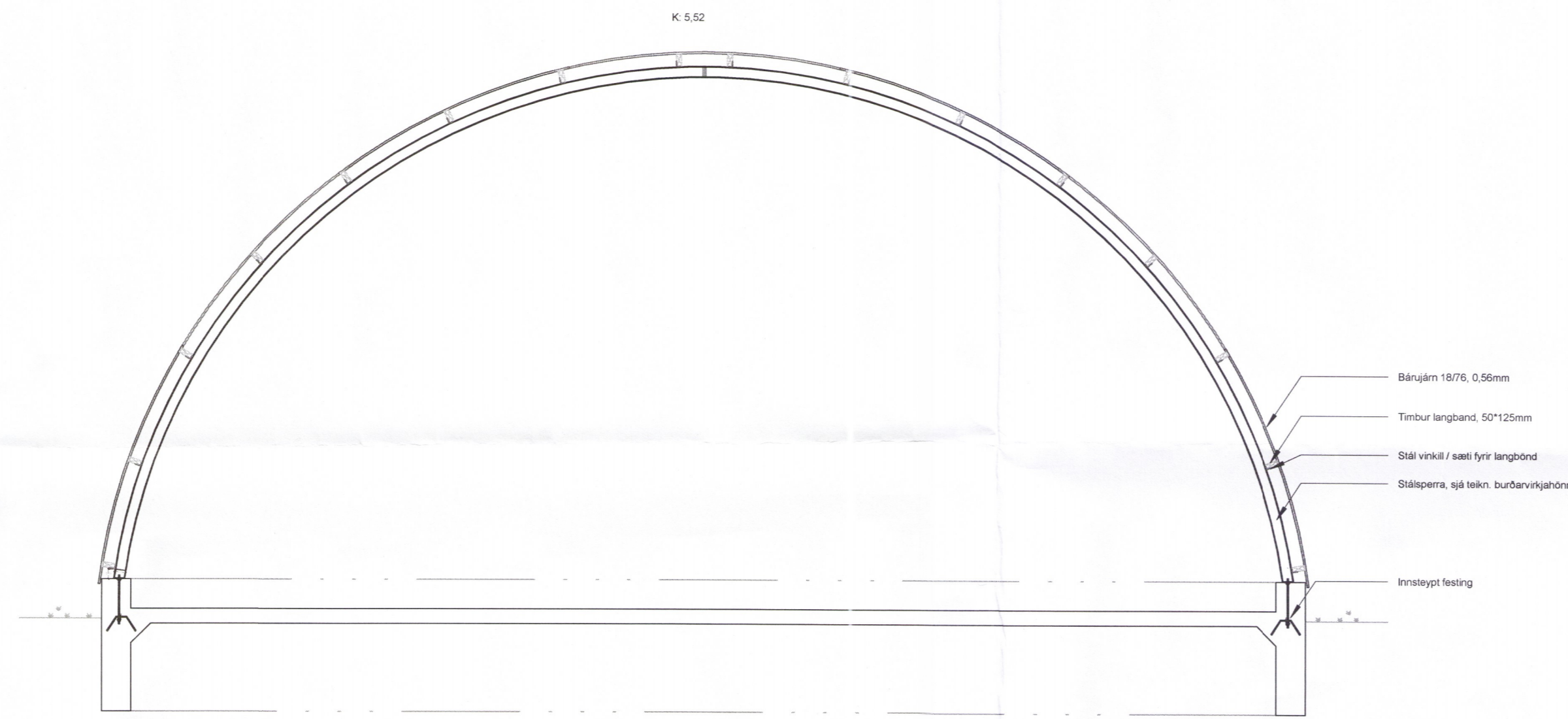
1 Snið 1 VT 1 : 50
