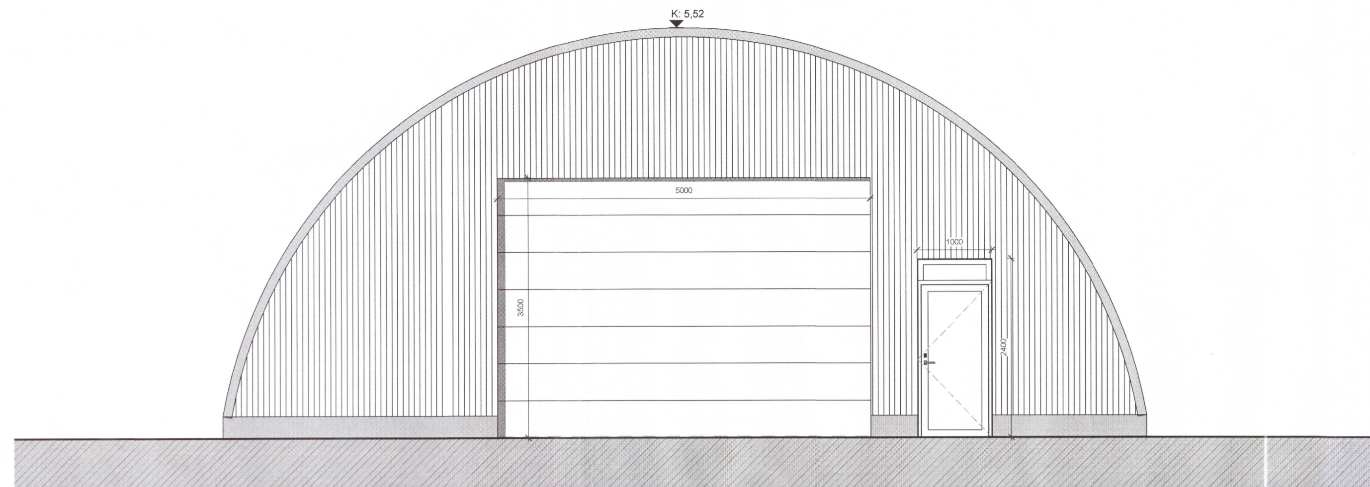
1 N-Austur VT 1 : 50
