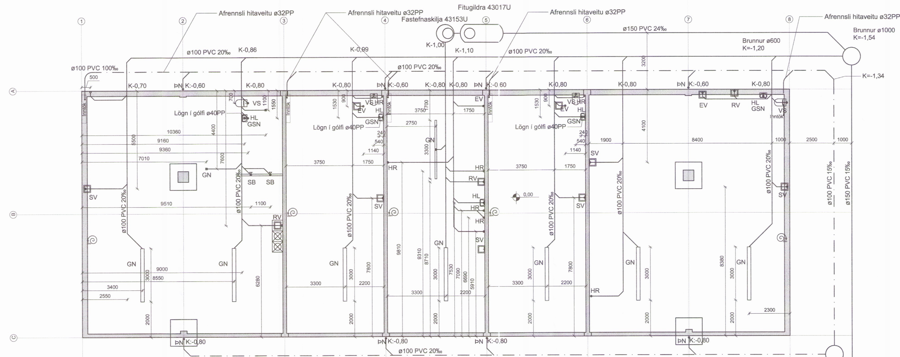
Frárennslislagir í grunni M 1:100
