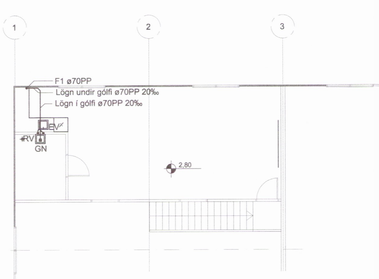
Frárennslislagir 2. hæð M 1:100
