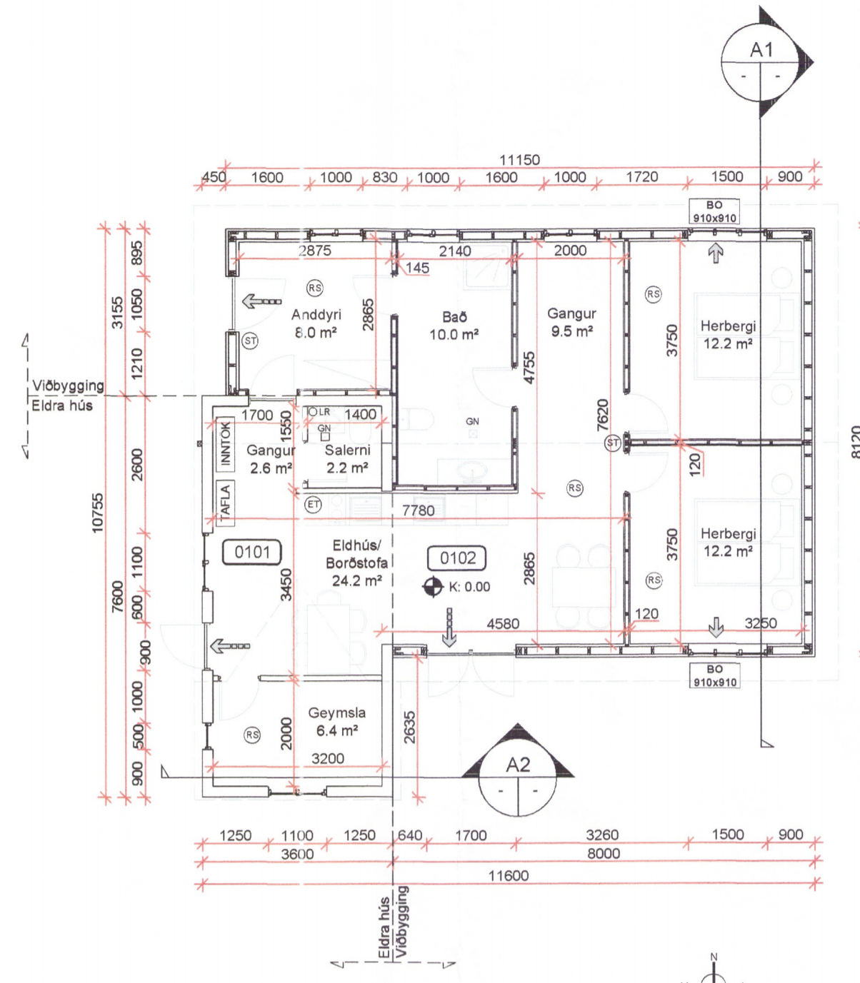
GRUNNMYND Mkv. 1:100
