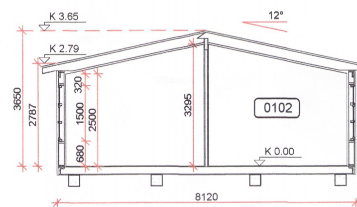
SNÍÐ A1 Mkv. 1:100
