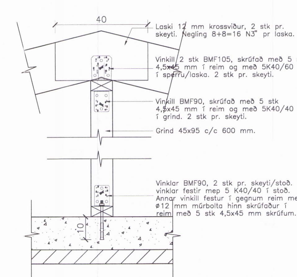
3.3 Sérmynd 3.3. 1:10.
