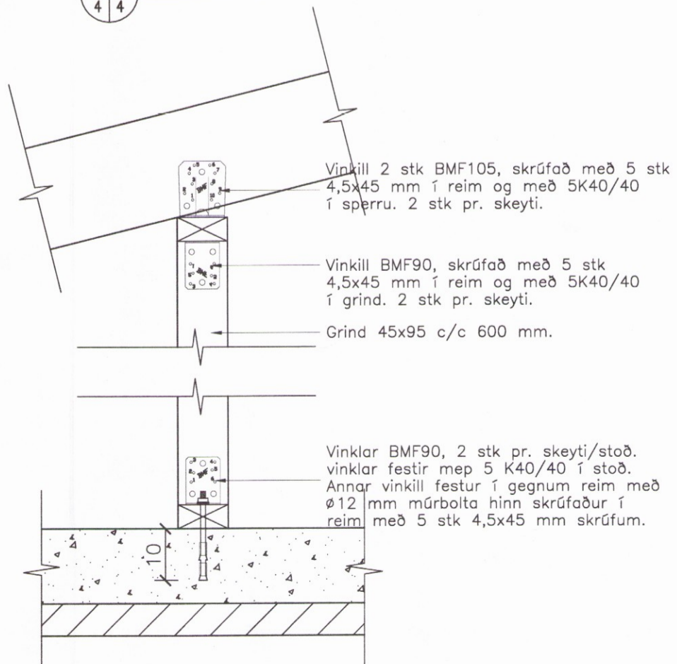
3.2 Sérmynd 3.2. 1:10.
