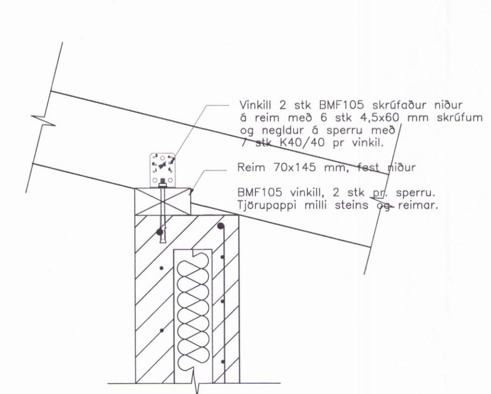
3.4 Sérmynd 3.4. 1:10.
