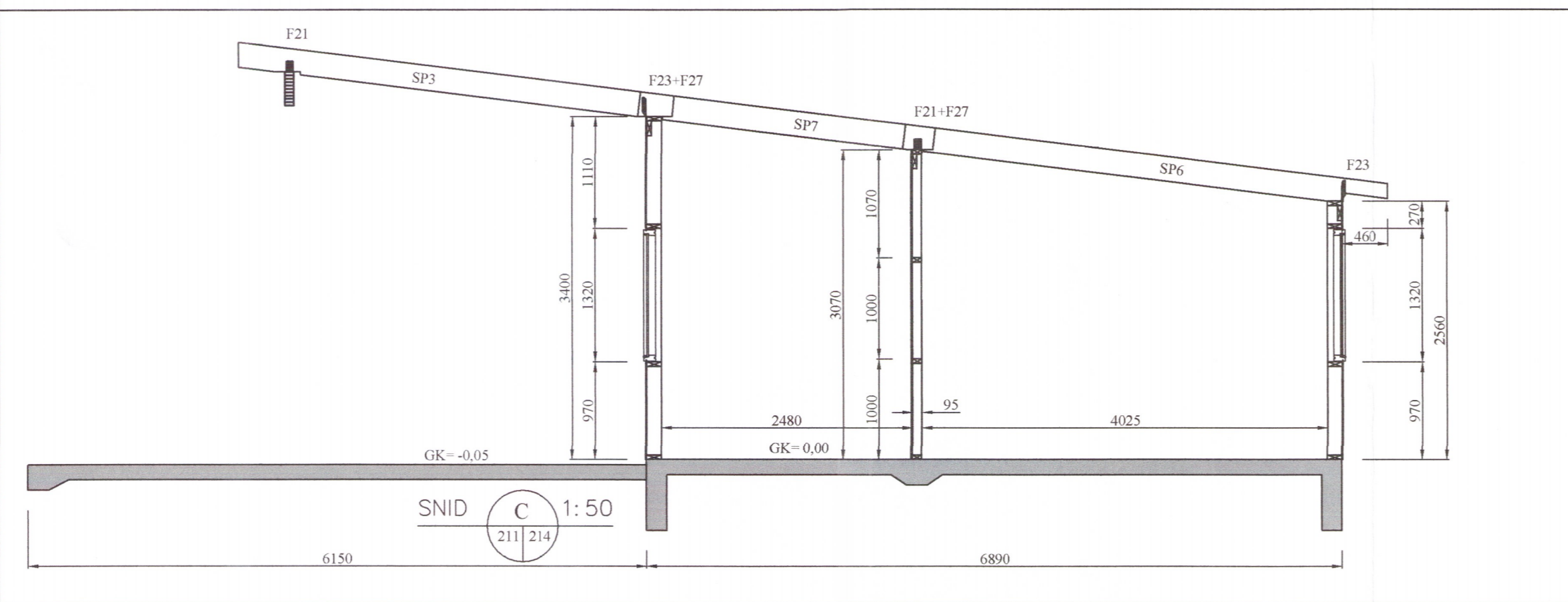
Snið í hús MKV. 1:50
