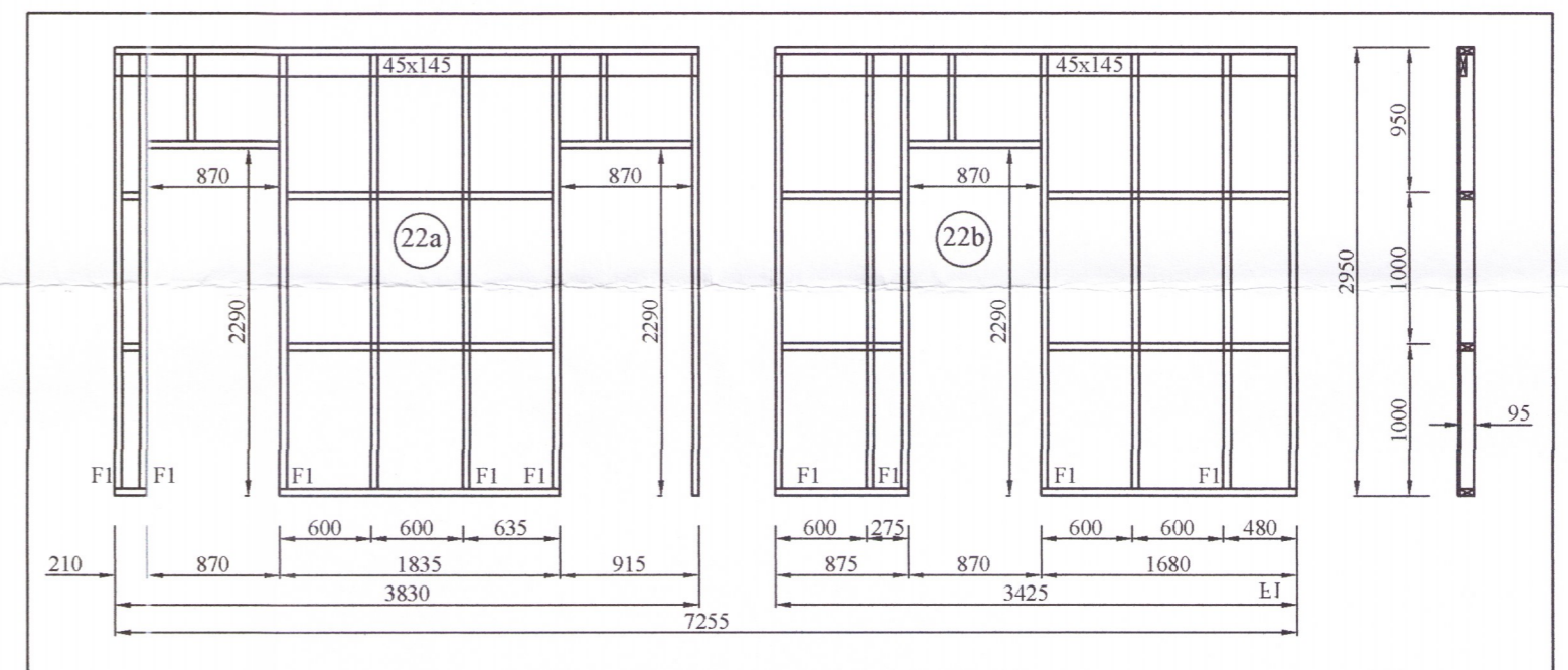
Innveggir, burðarveggir MKV. 1:50
