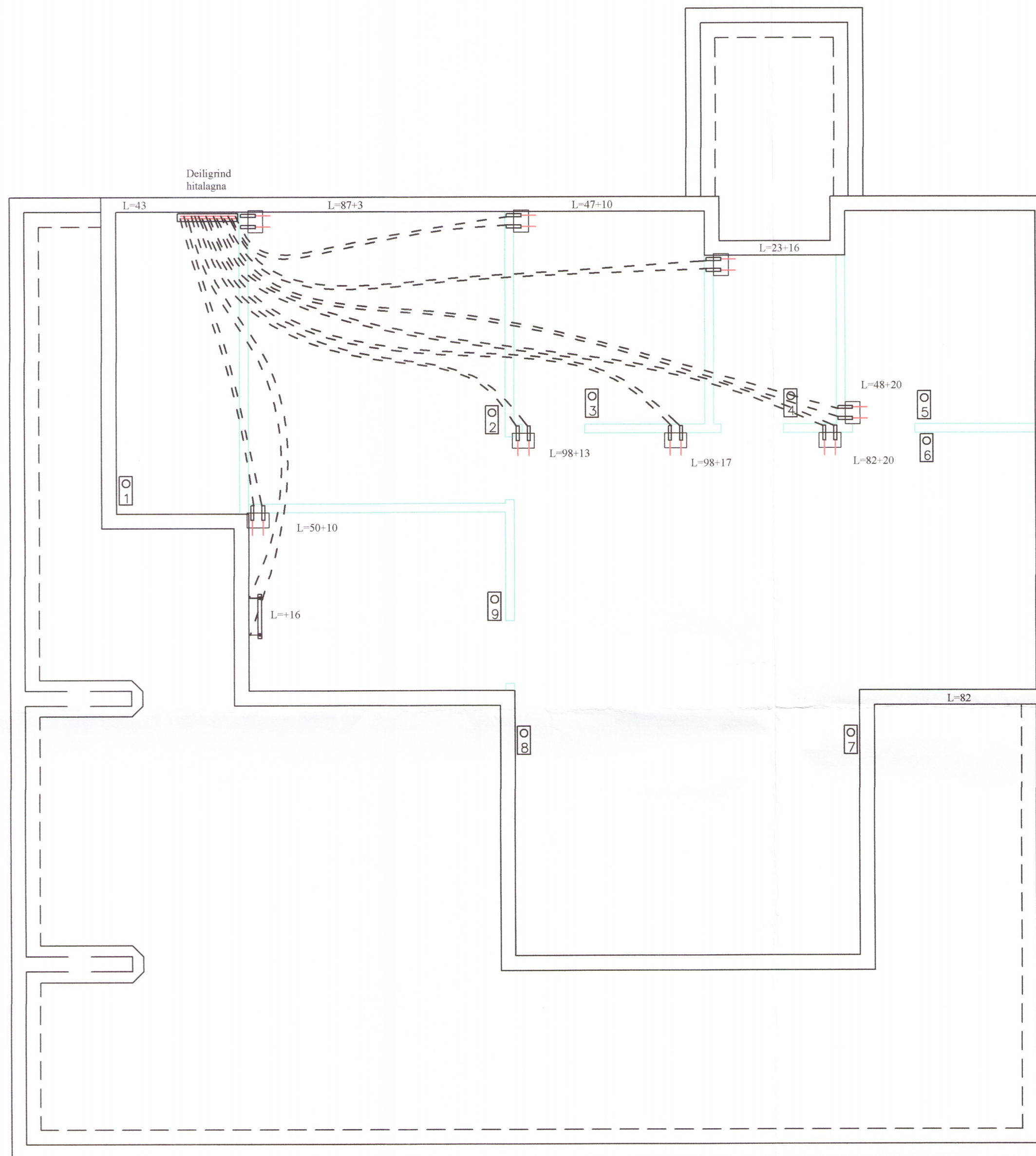
Grunnmynd idráttalagna fyrir heitavatslagnir MKV: 1:50
