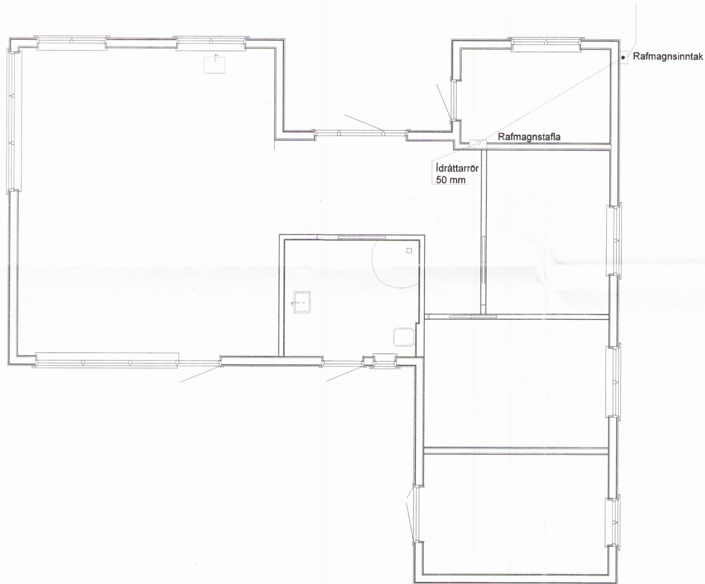
Grunnmynd hús, rafmagnsinntak og tafla 1 : 50
