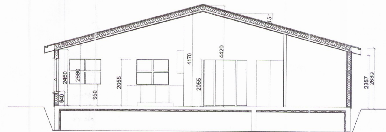
Snið A - A
