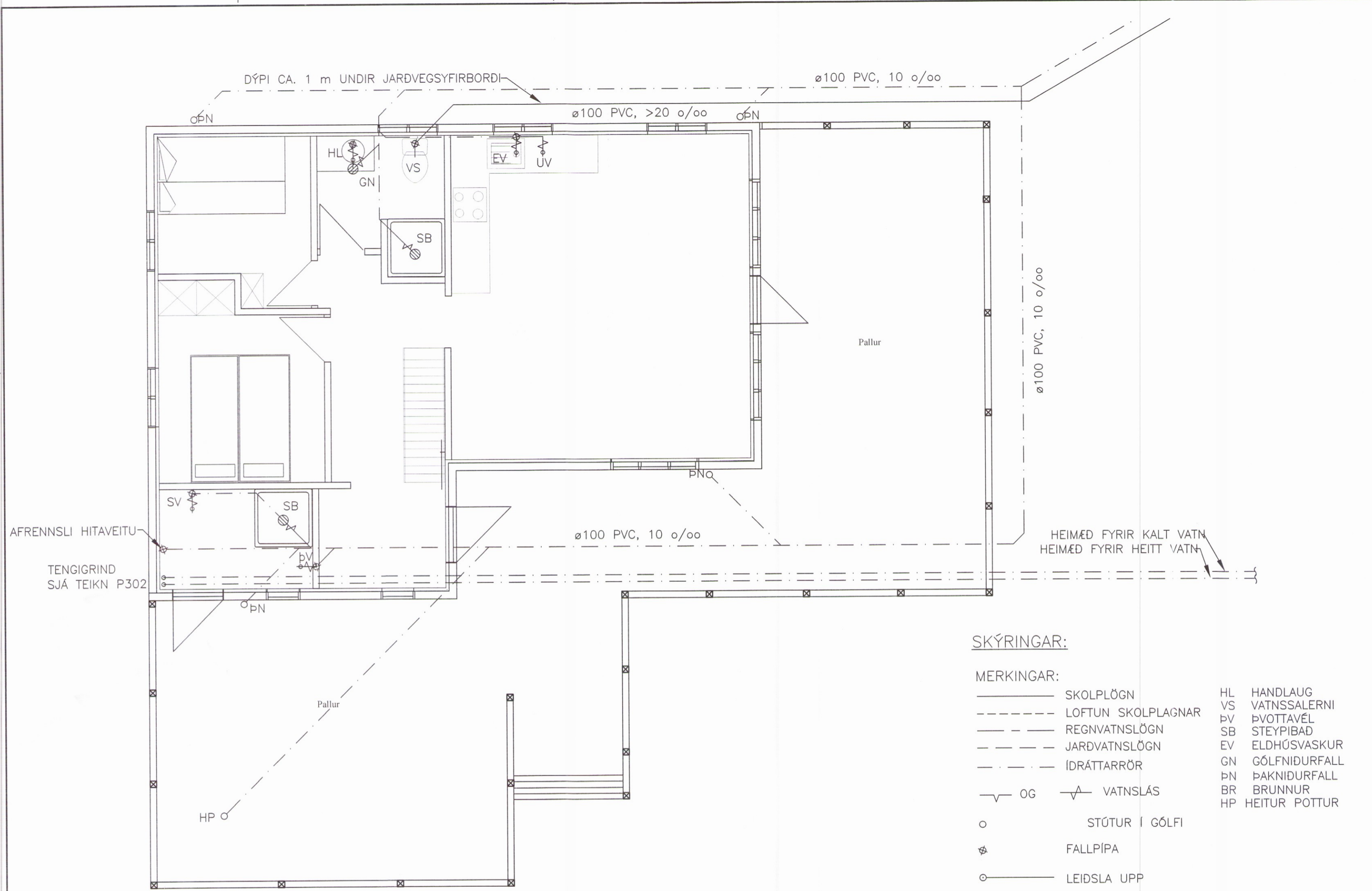
GRUNNMYND 1:50
