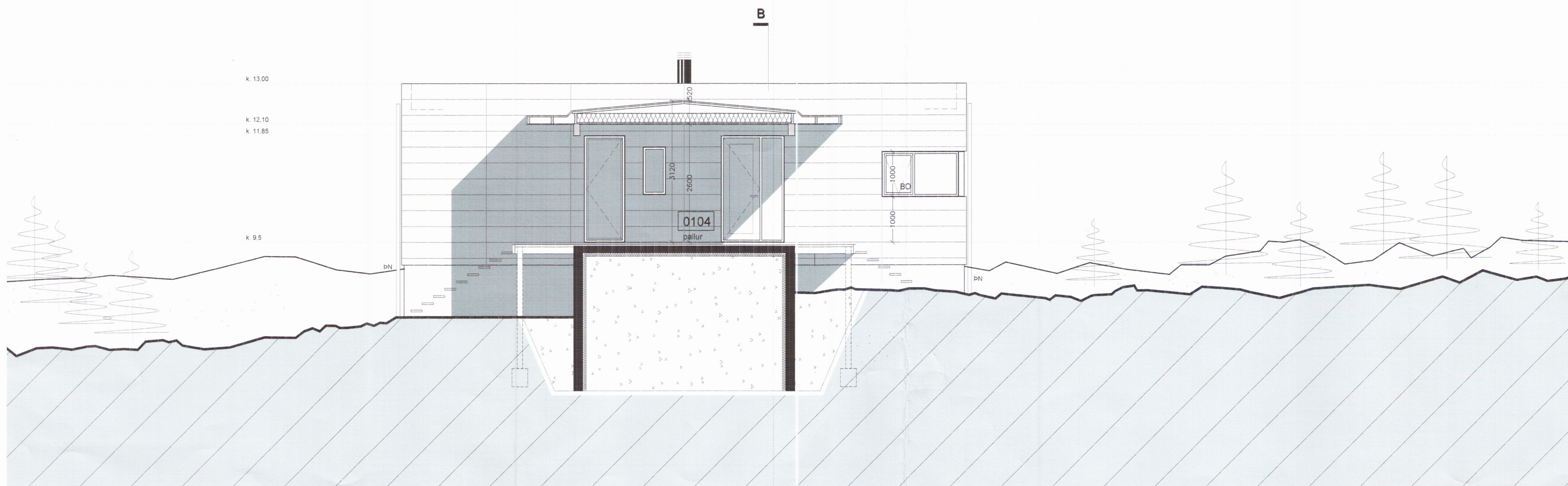
SNEIÐING D - D M 1:50
