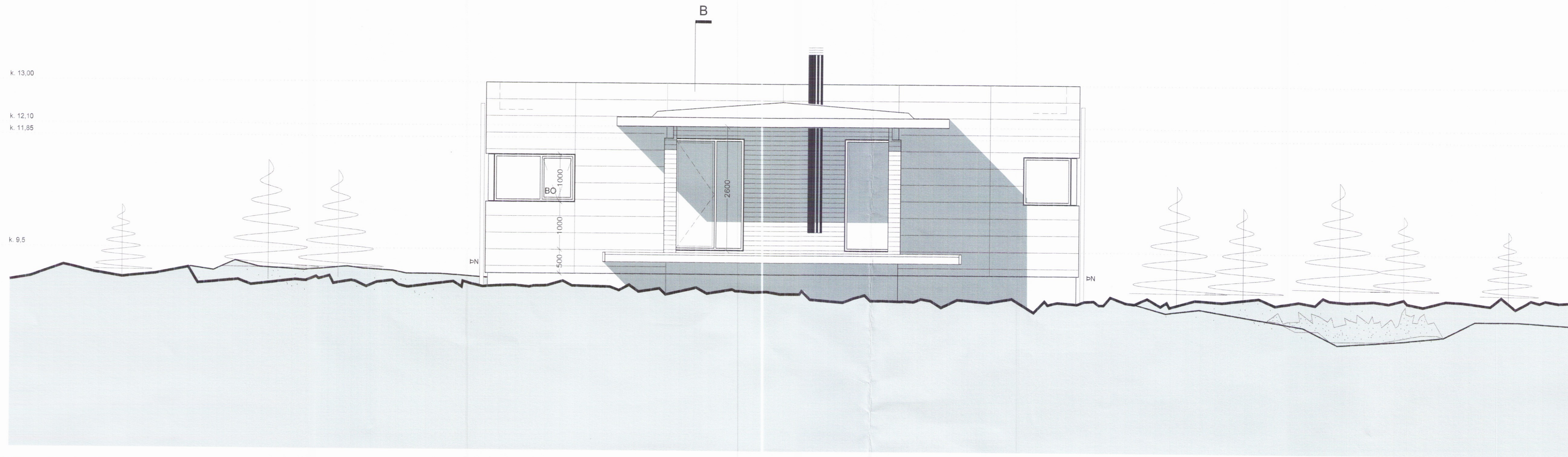
ÚTLIT SUÐUR M 1 : 50
