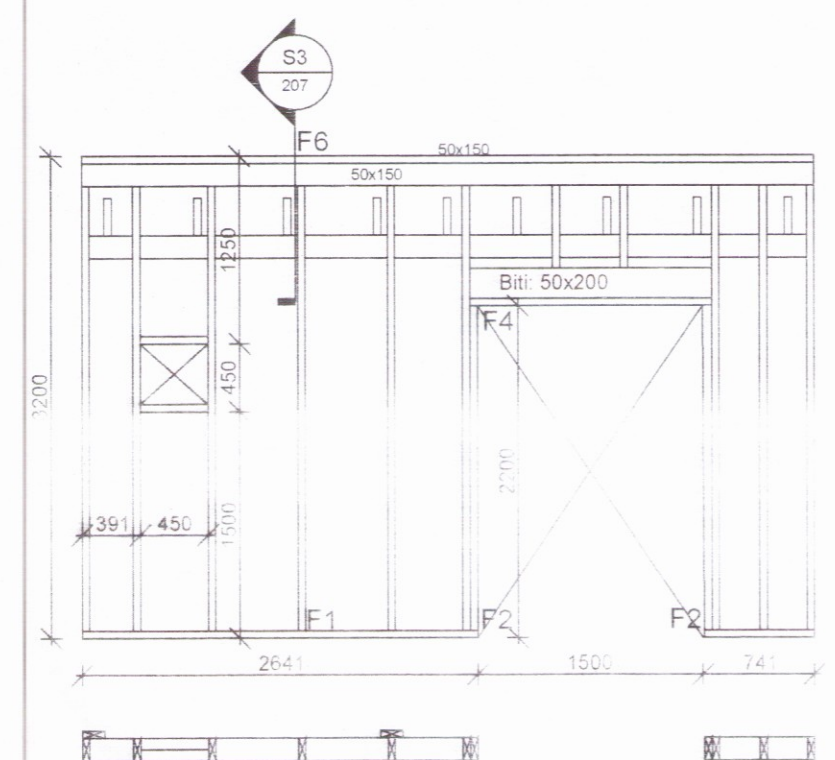
U6 Útbýgging - grind 1:50
