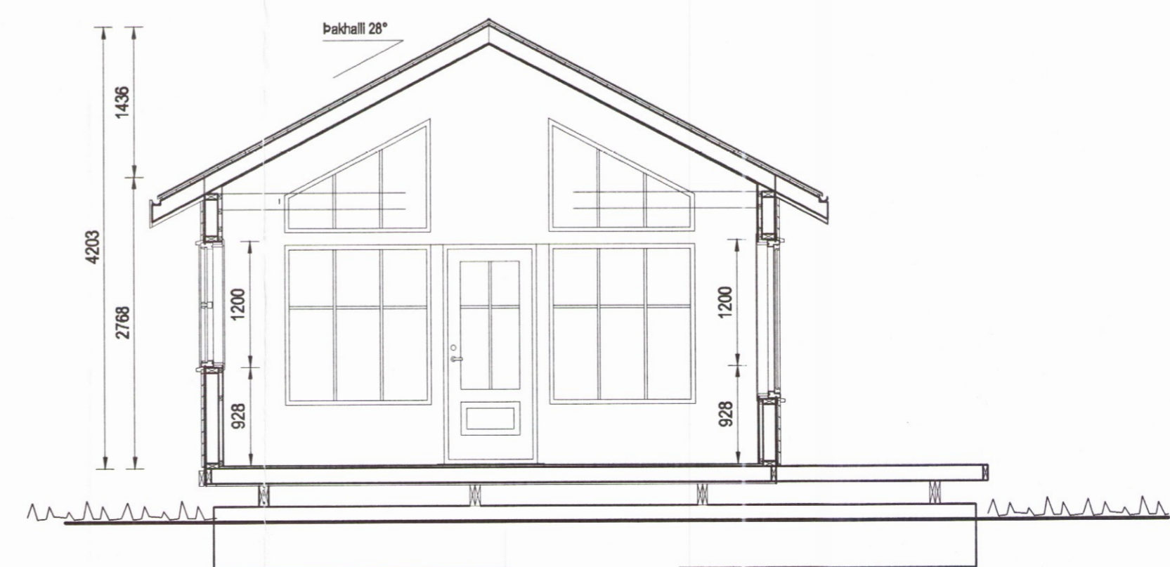
SNÍÐ A-A
