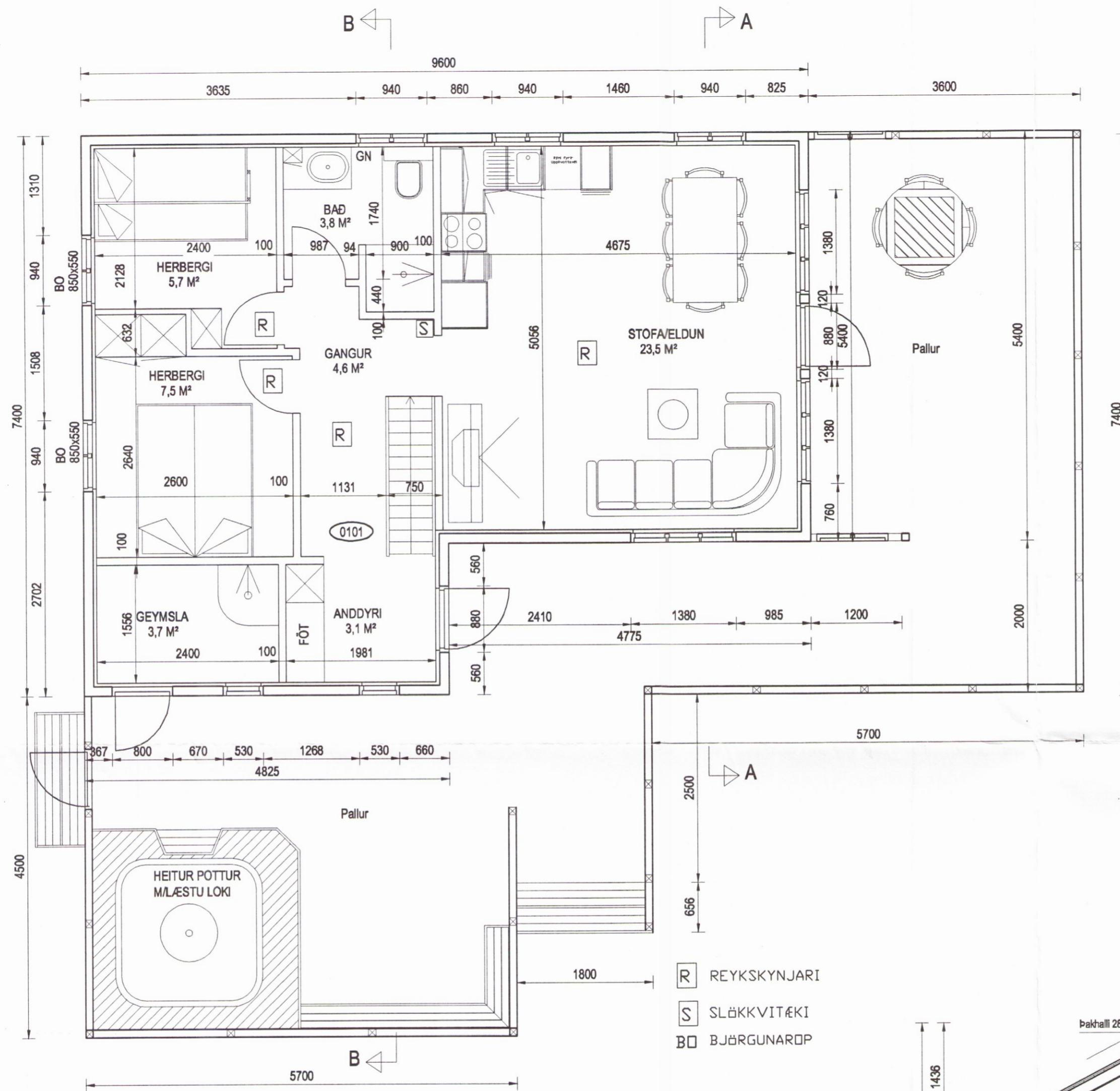
GRUNNMYND MKV. 1:50
