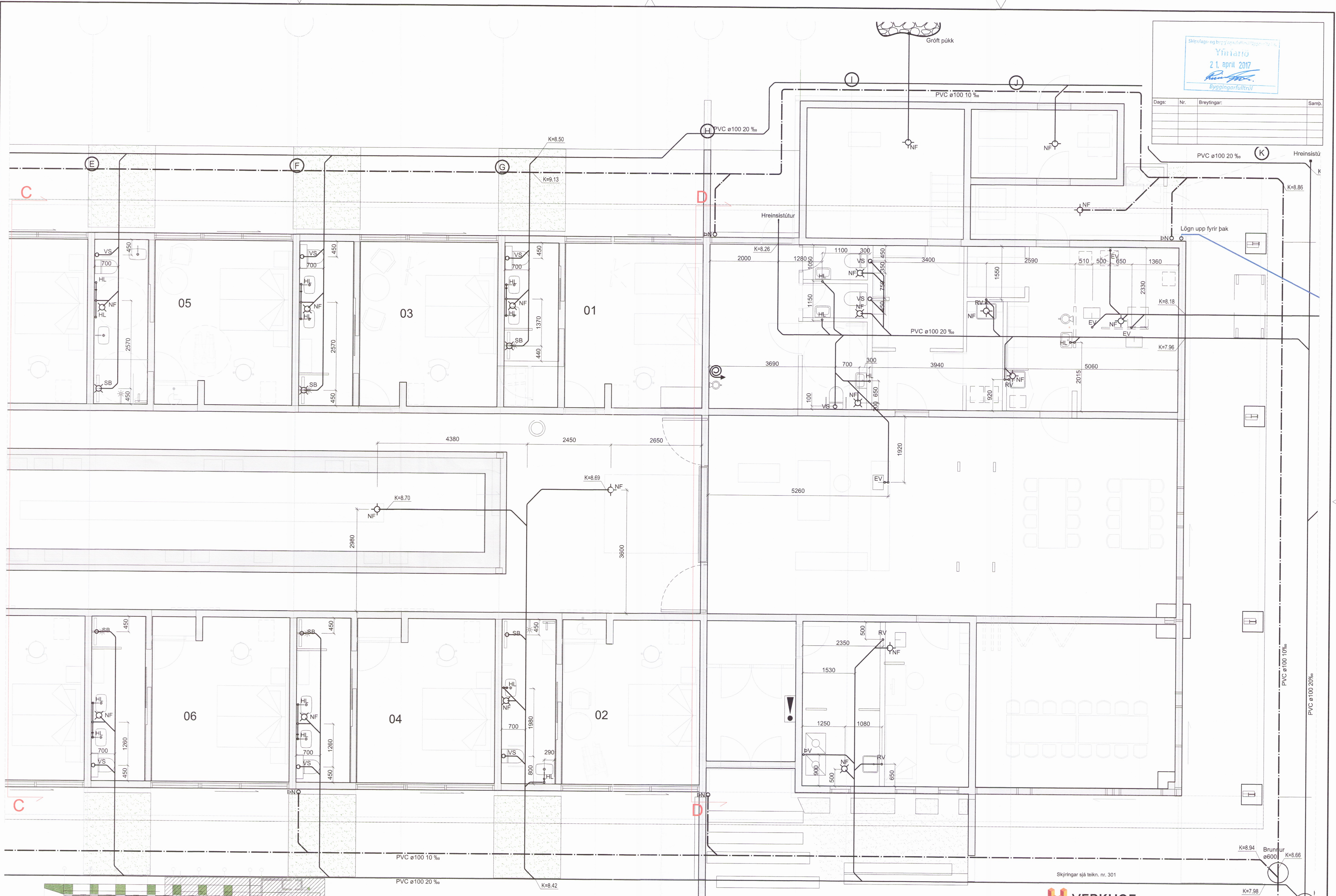
Grunnmynd - 1. hæð Mkv. 1:50
