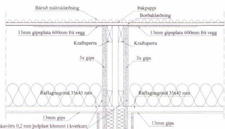
Lóðrétt sneið í útvegg mkv. 1:20
