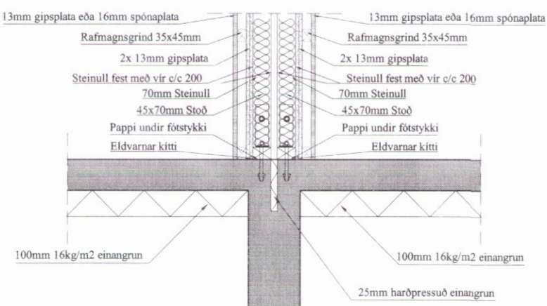
Lóðrétt sneið í millivegg (fóstystykki) milli íbúða E190
