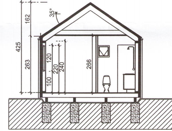
Snið A-A 1:100
