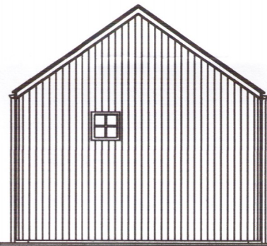
Norðausturhlið 1:100
