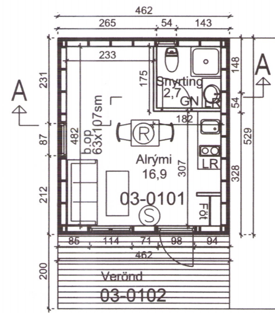
Grunnmynd 1:100
