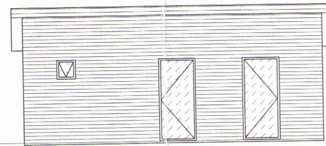
Útlit gesthús austur 1:100
