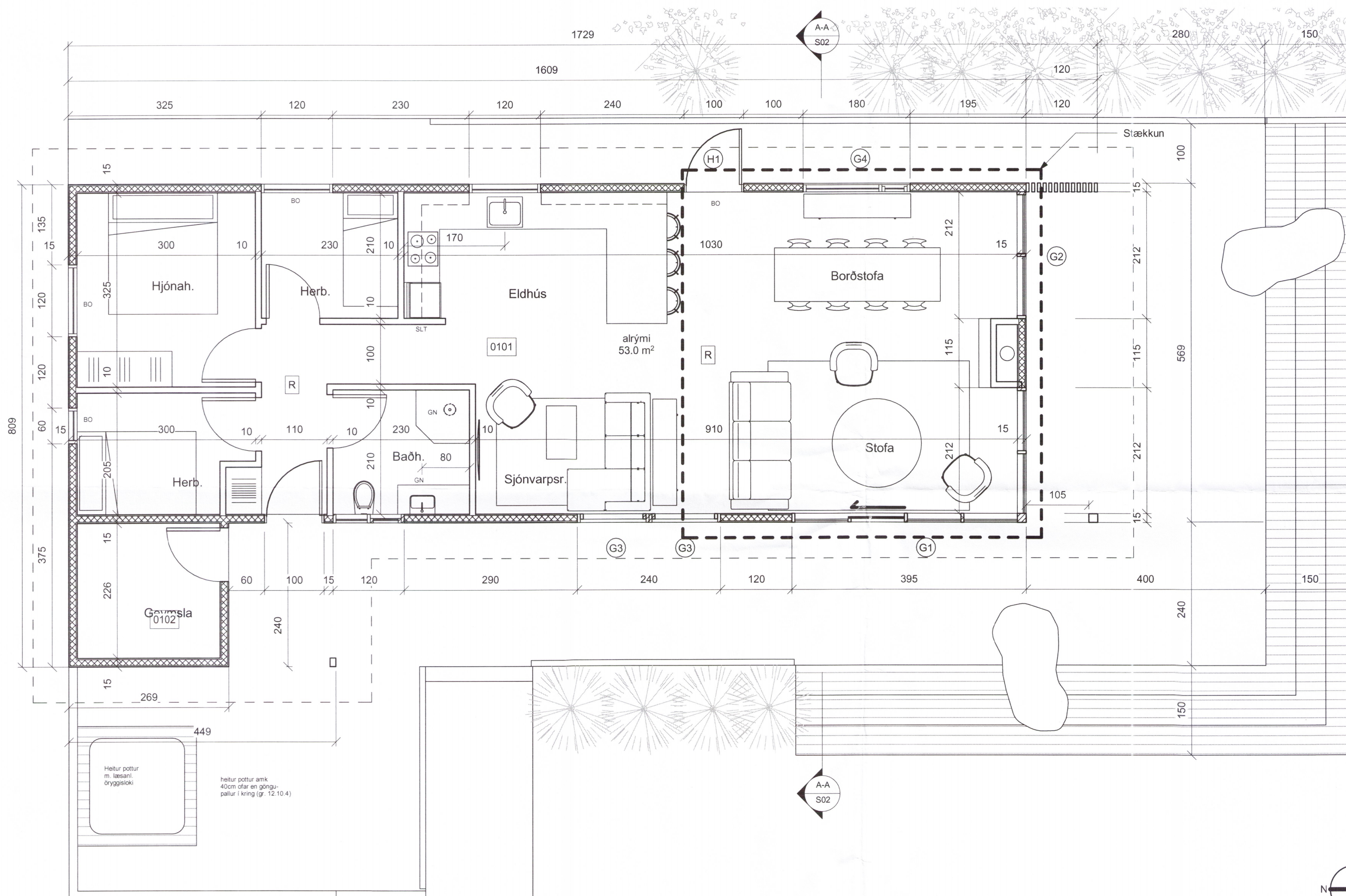
Grunnmynd 1-50 1 : 50
