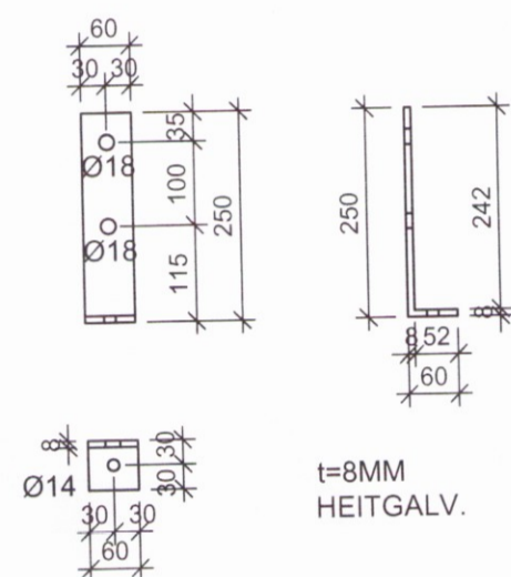
F1 FESTIJÄRN 05 Mkv. 1/10 3. stk
