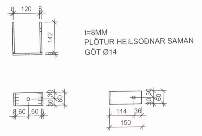
F7 FESTIJÄRN 05 Mkv. 1/10 1. stk
