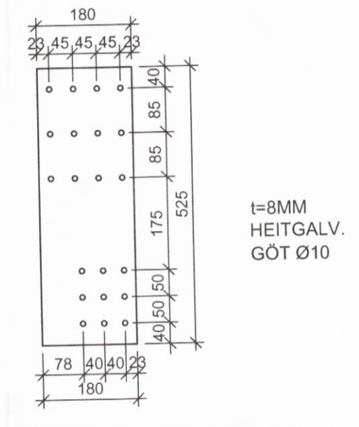
F3 FESTIJÄRN 05 Mkv. 1/10 1. stk
