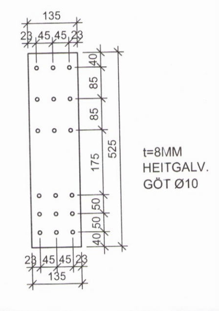
F4 FESTIJÄRN 05 Mkv. 1/10 1. stk
