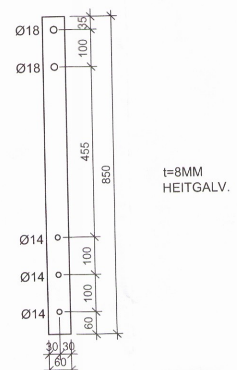
F2 FESTIJÄRN 05 Mkv. 1/10 1. stk
