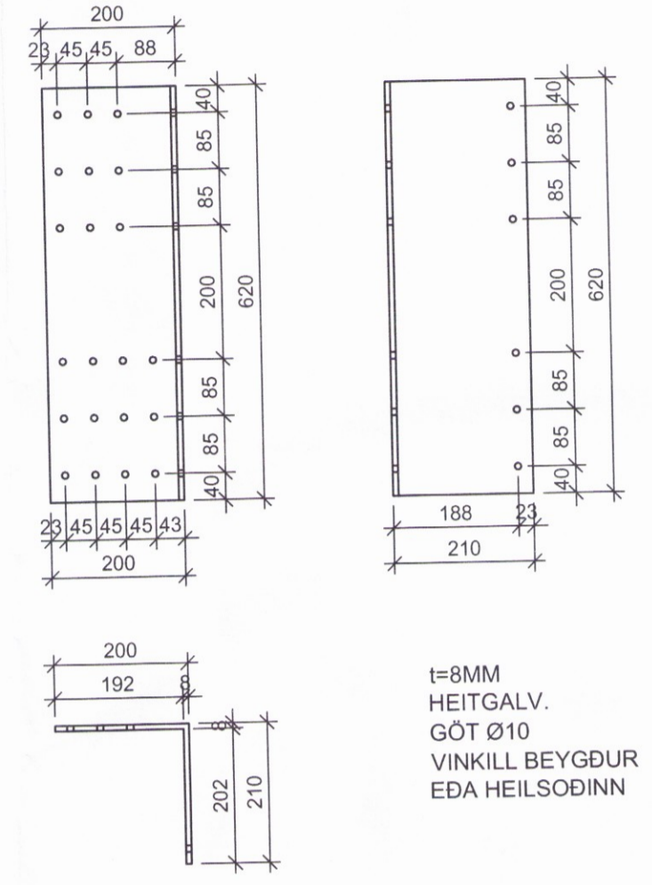
F5 FESTIJÄRN 05 Mkv. 1/10 1. stk
