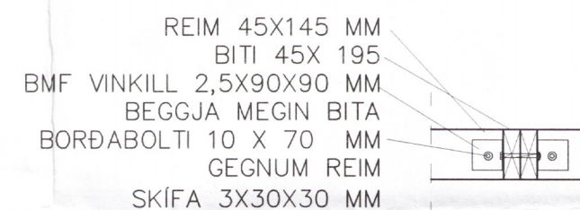
SNID 7 MILLIGÓLF-INNVEGG
