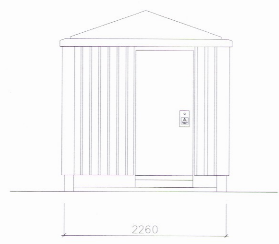
NORÐVESTUR GAFL
