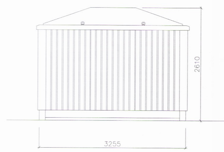
HLÍÐAR
