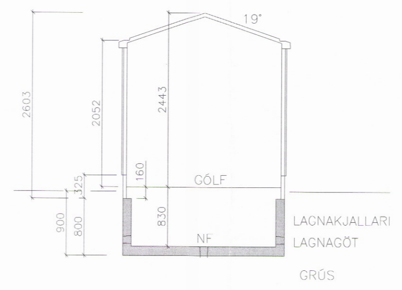
SNÍÐ
