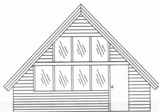
Útlit vestur mkv: 1:100
