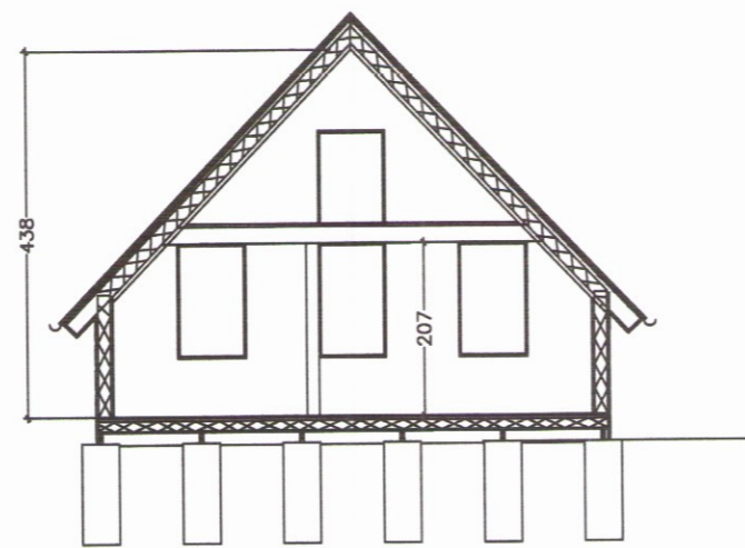
Snið A-A mkv: 1:100
