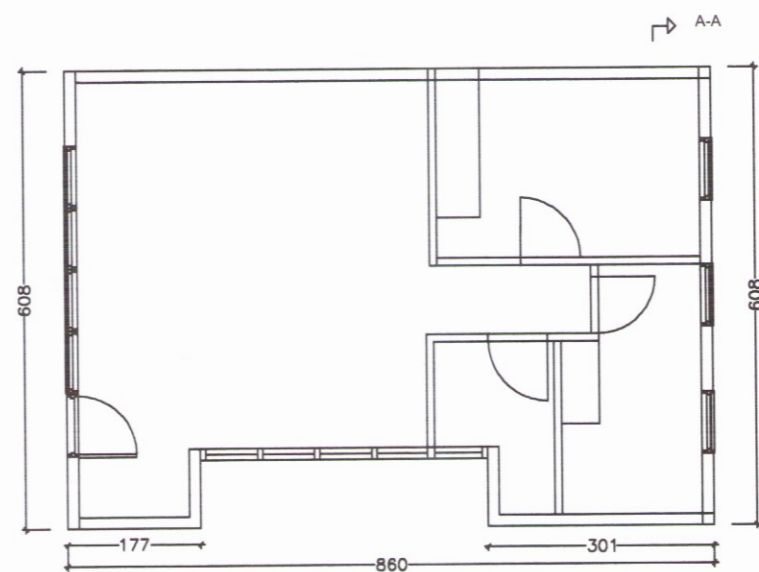
Grunnmynd mkv: 1:100
