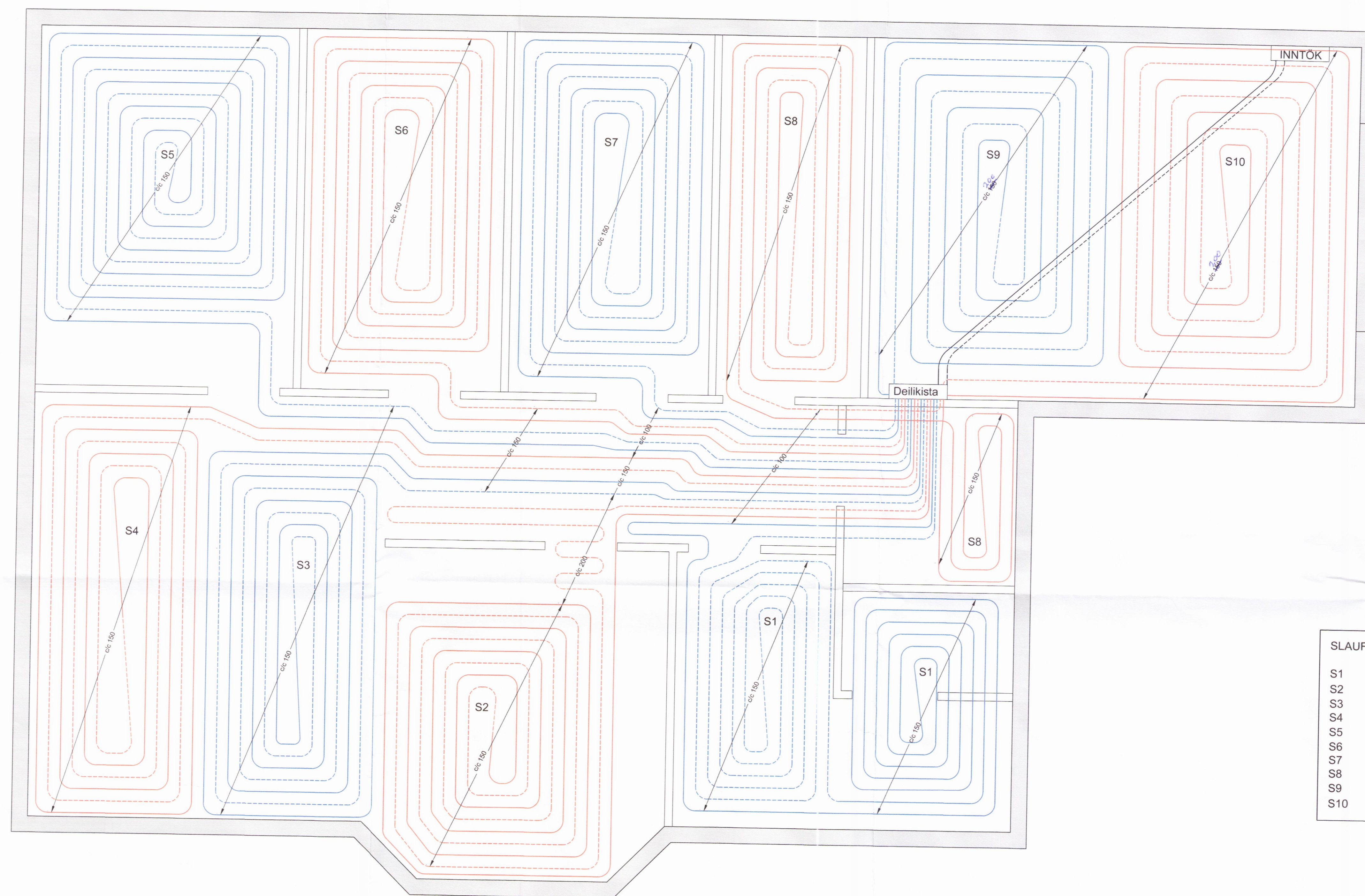
GRUNNMYND HITALAGNIR MKV. 1:30
