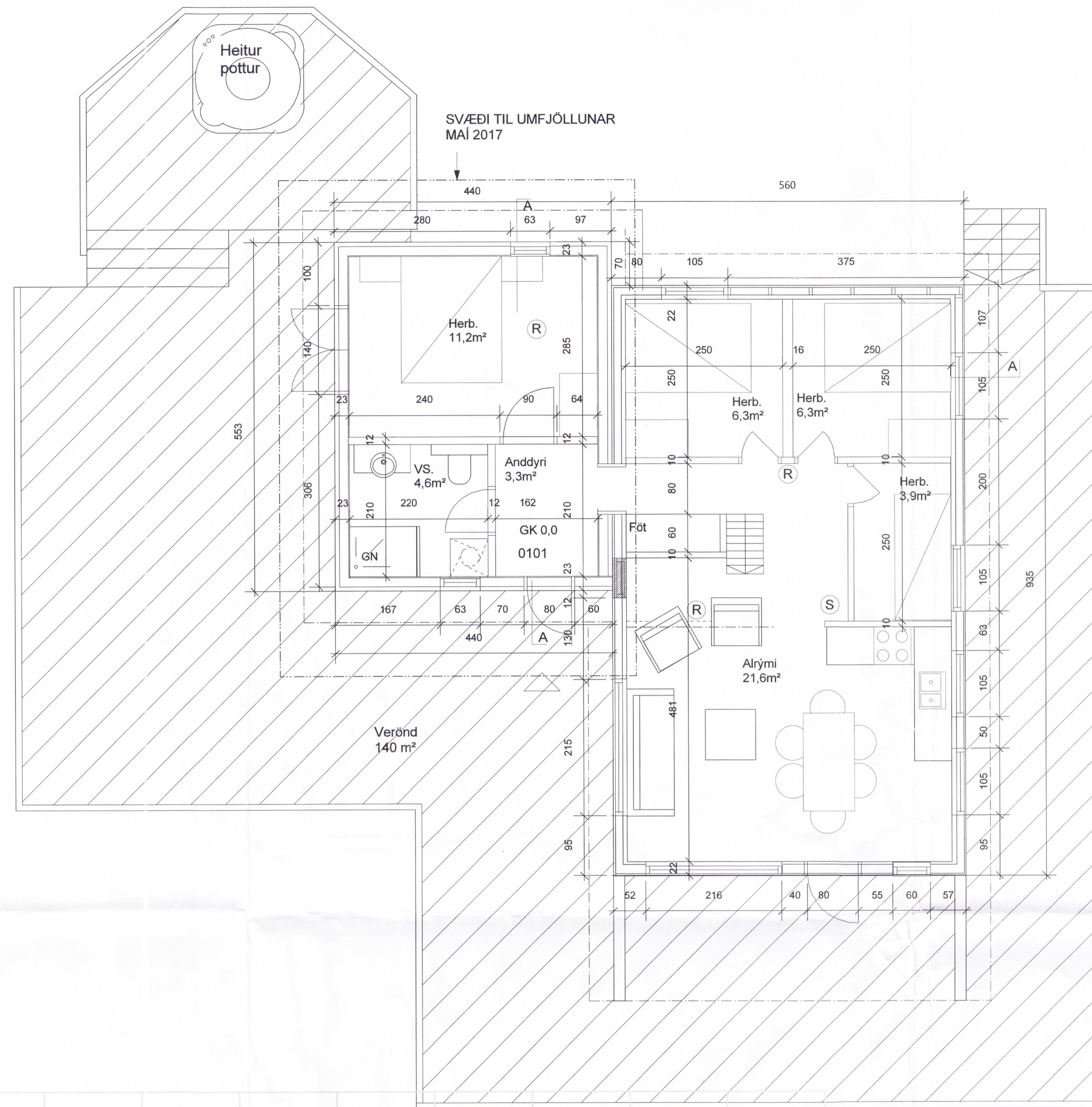
GRUNNMYND 1:50
