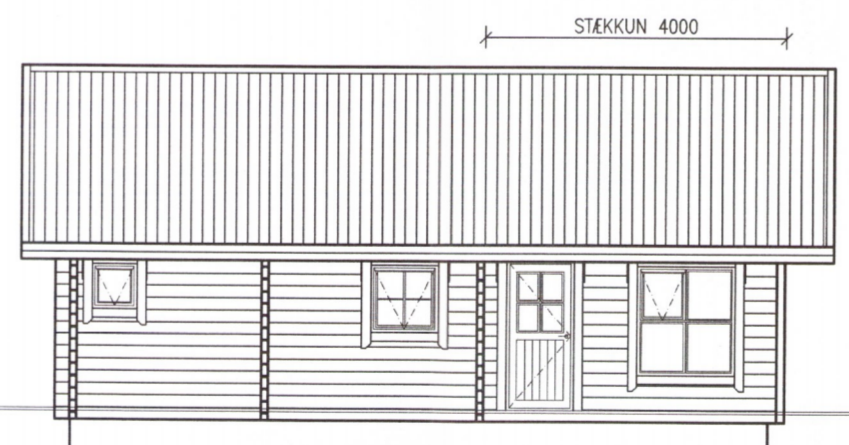
ÚTLIT VESTURHLIÐ
