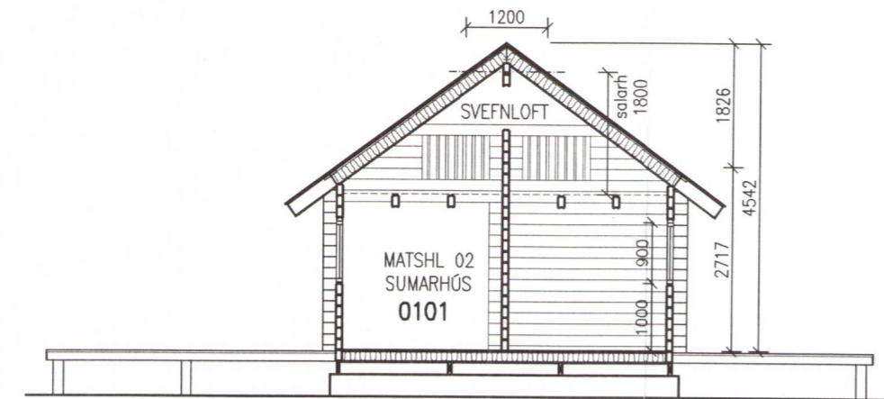
SNID 1-1 1:100
