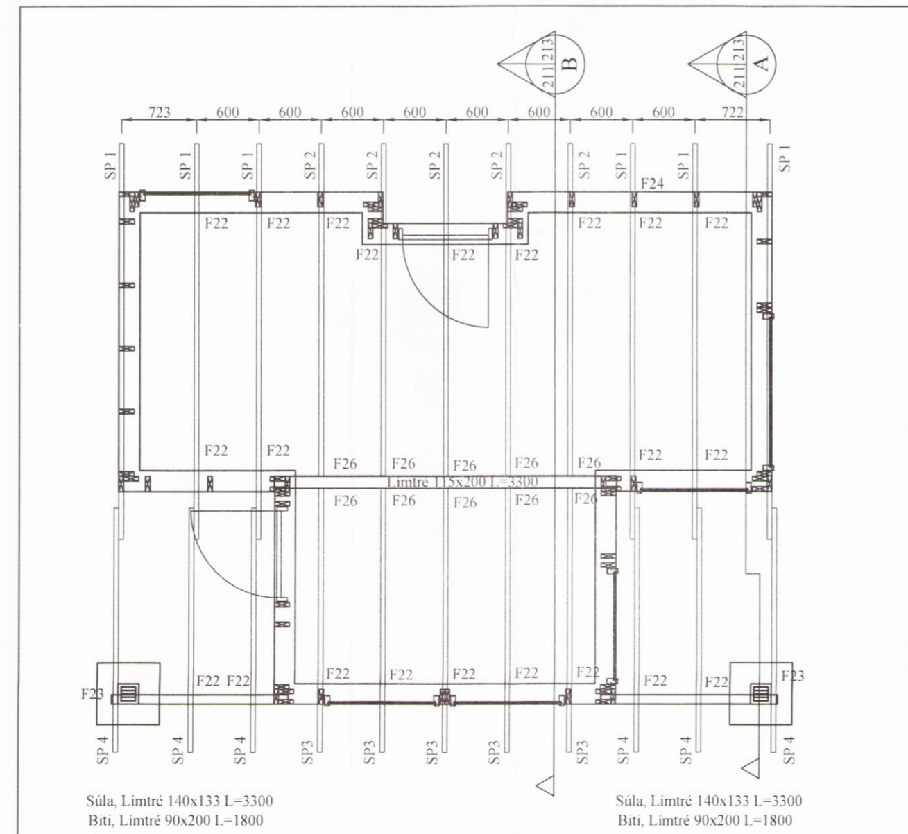
Grunnmynd þarkplans MKV. 1:50
