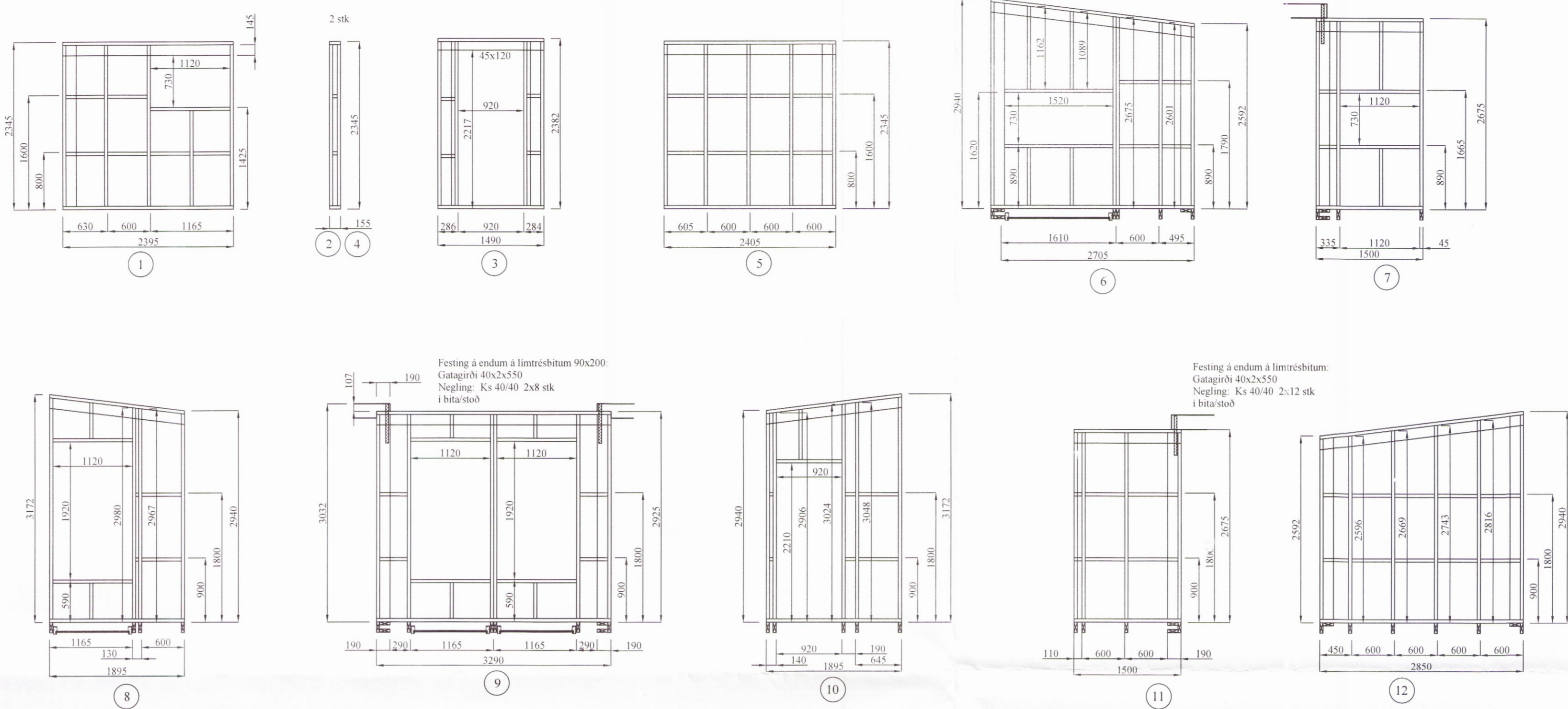
Útveggir séðir utanfrá MKV. 1:50
