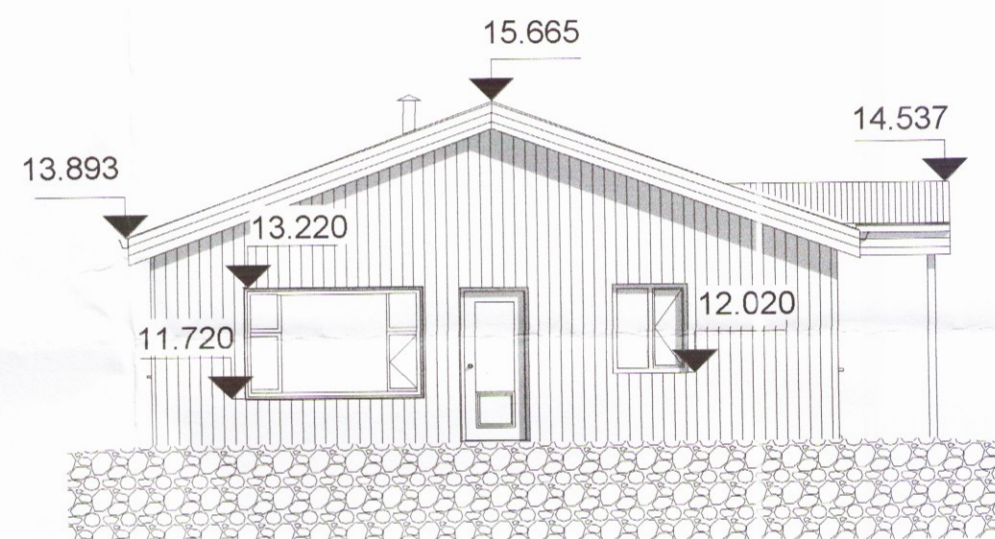
Suður Aðalupp útlit 1 : 100
