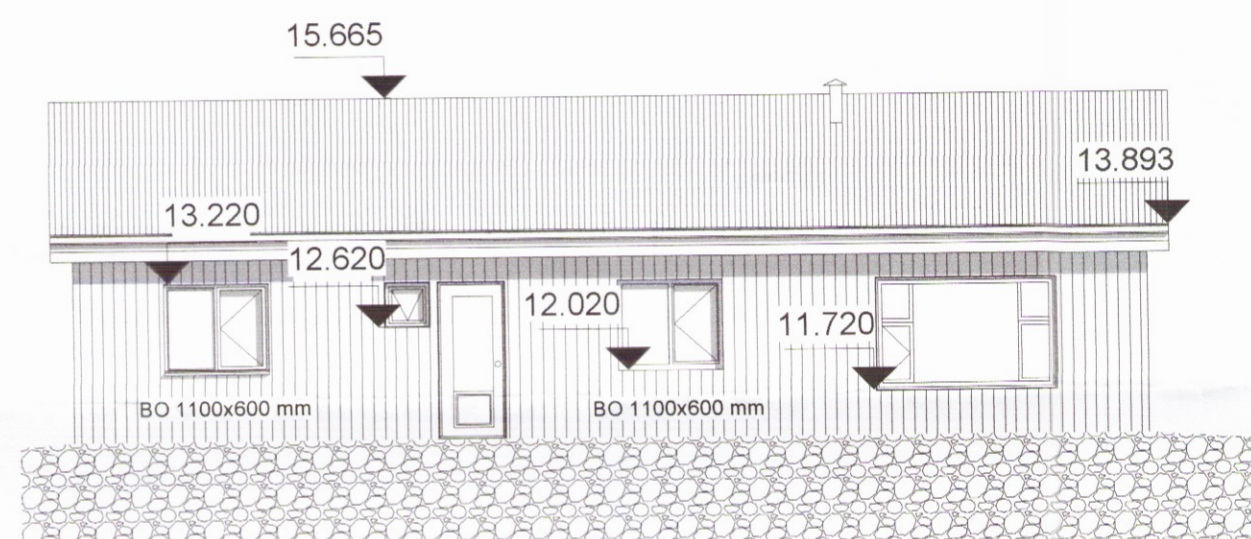
Vestur Aðalupp útlit 1 : 100
