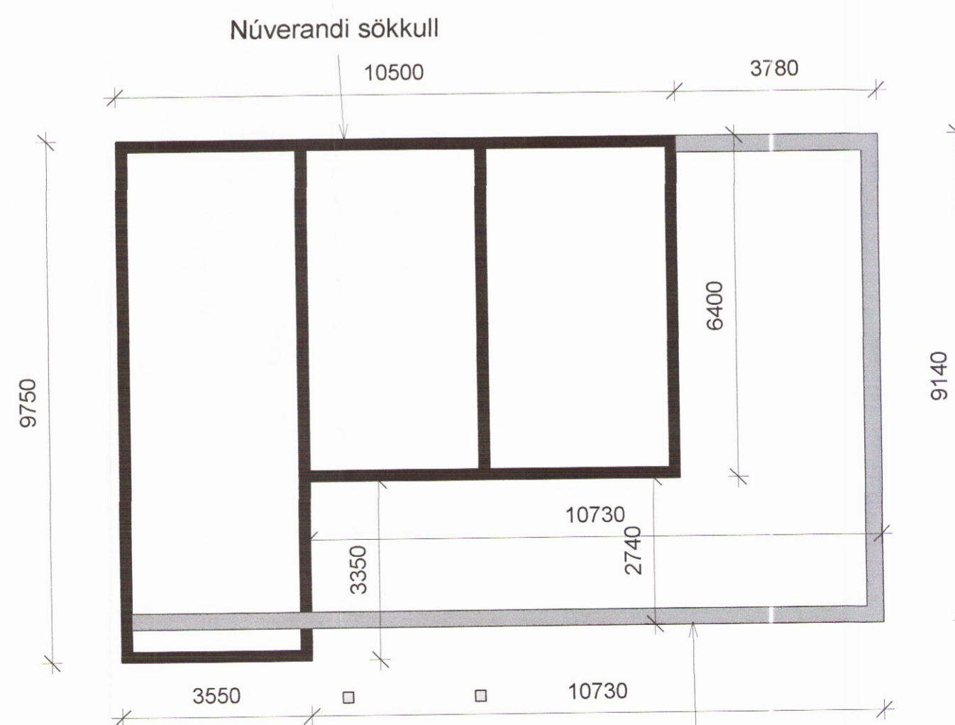
00 Sökkulteikning 1 : 100
