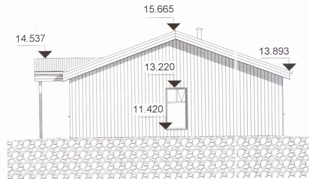
Norður Aðalupp útlit 1 : 100
