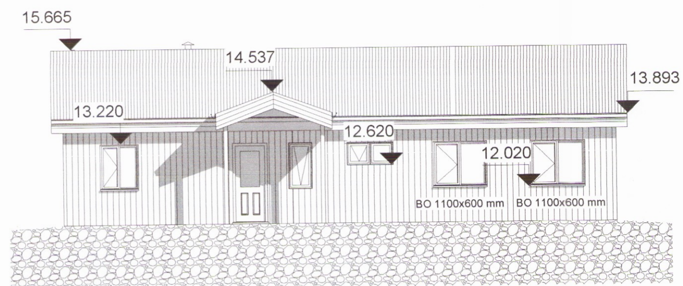
Austur Aðalupp útlit 1 : 100
