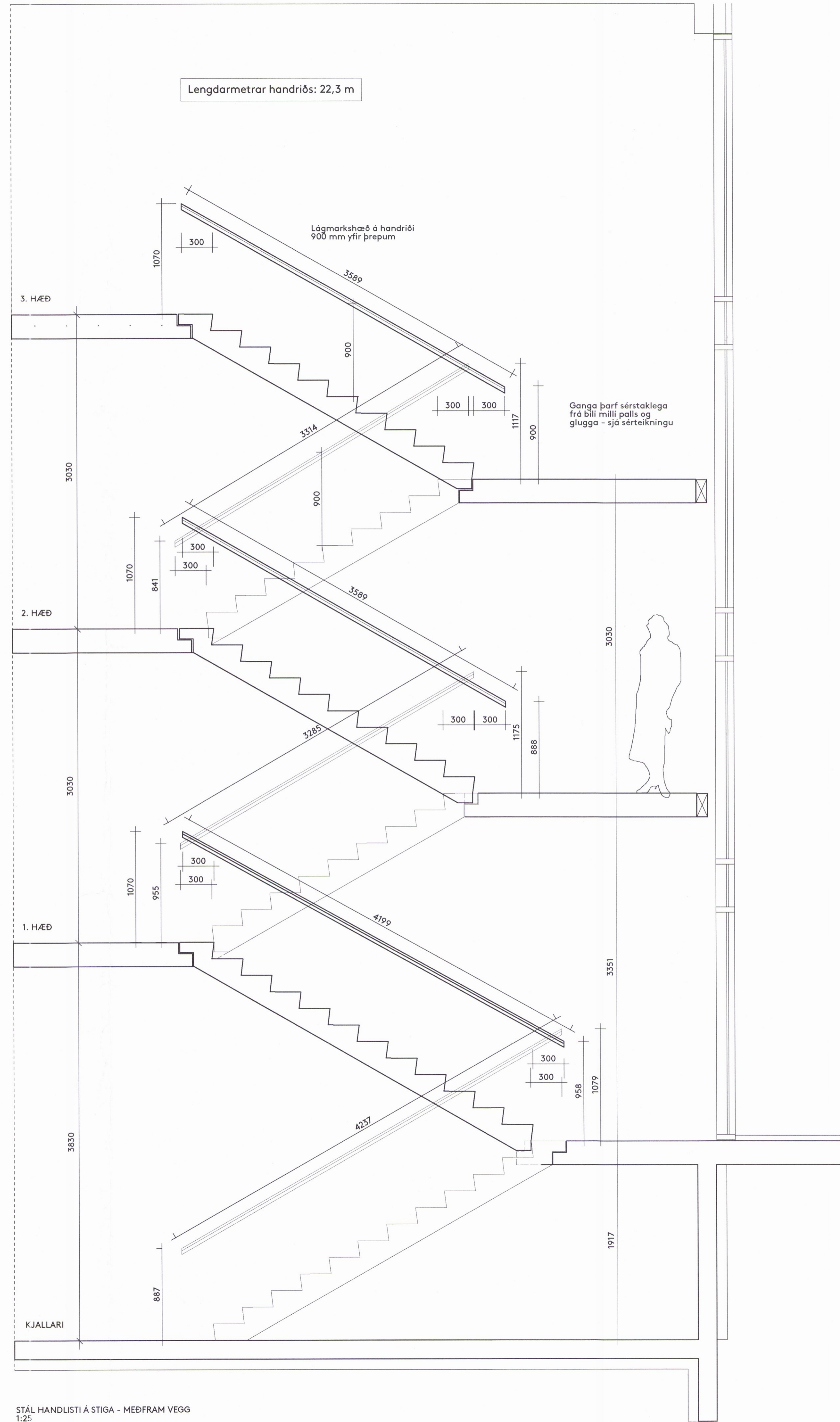
STÁL HANDLISTI Á STIGA - MEÐFRAM VEGG 1:25
