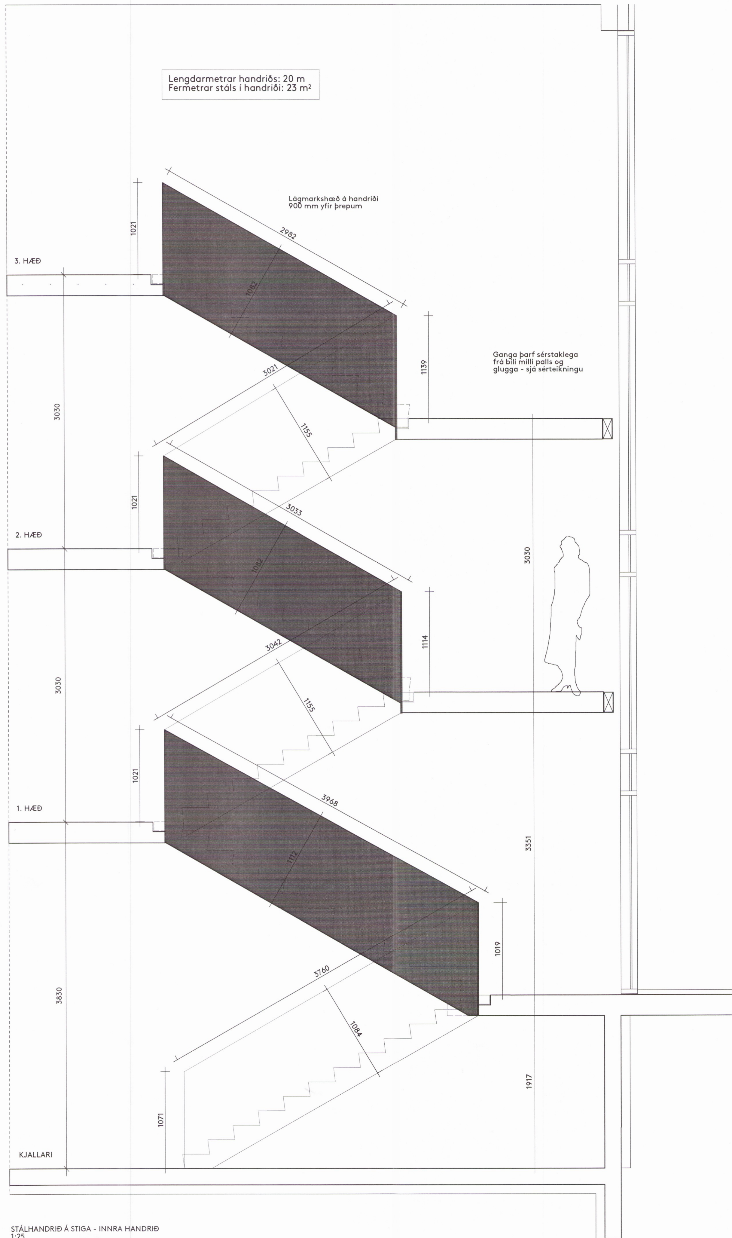
STÁLHANDRIÐ Á STIGA - INNRA HANDRIÐ 1:25
