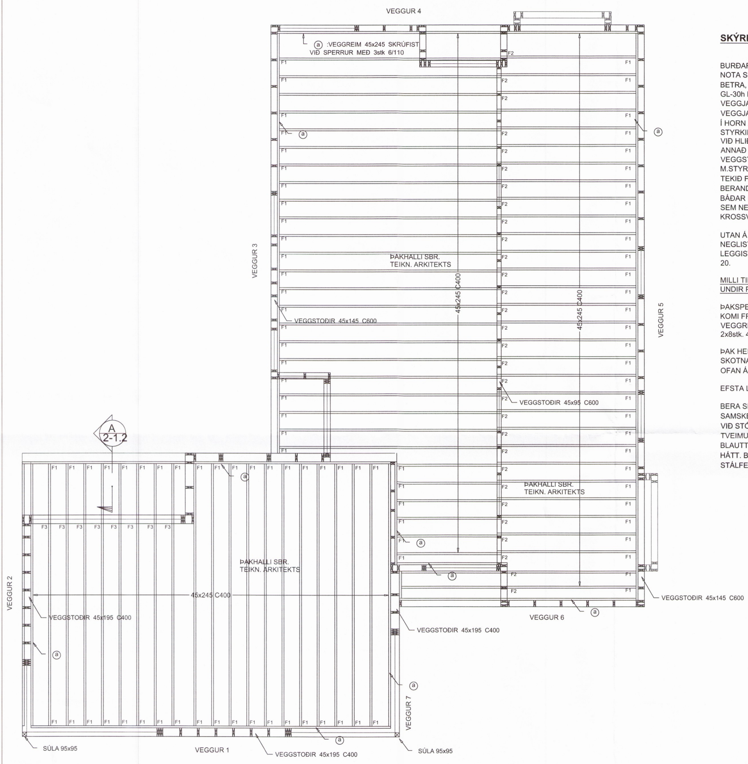
GRUNNMYND ÞAKS 1:50
