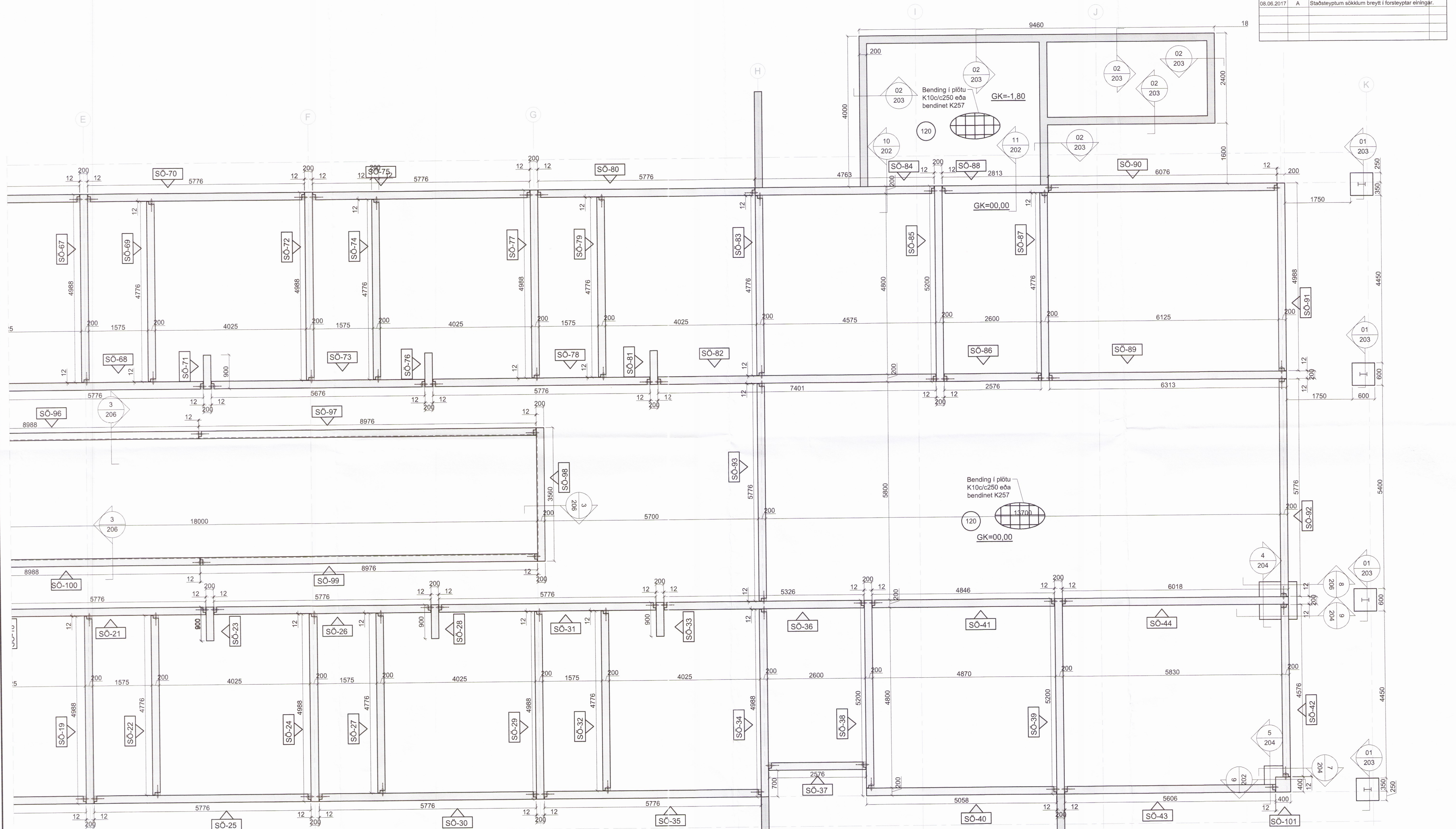
Grunnmynd sökkla Mkv. 1:50
