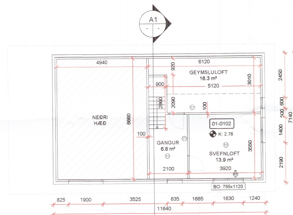
GRUNNMYND SVEFNLOFT Mkv. 1:100
