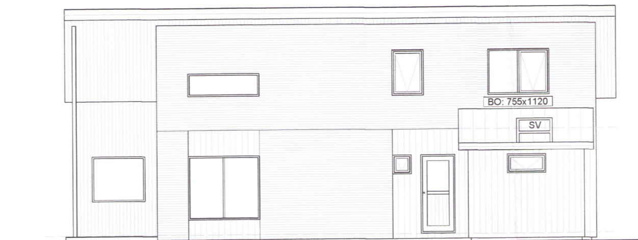
ÚTLIT SUÐUR Mkv. 1:100
