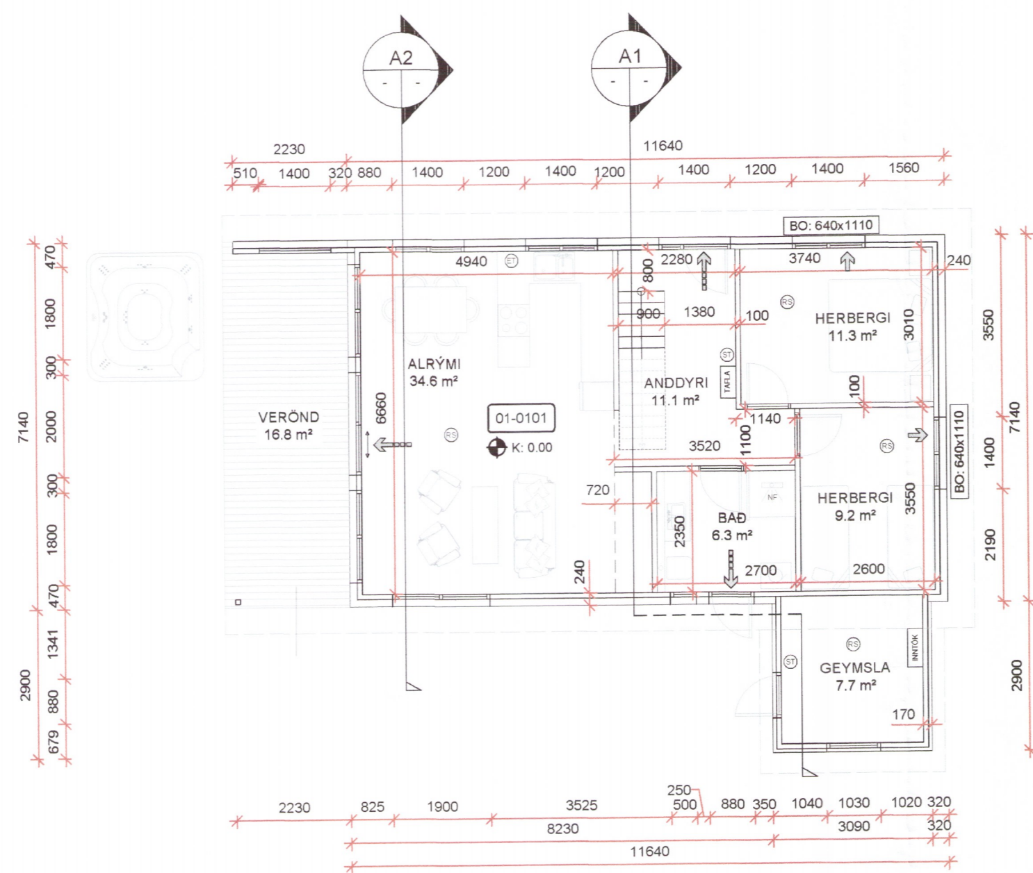
GRUNNMYND Mkv. 1:100
