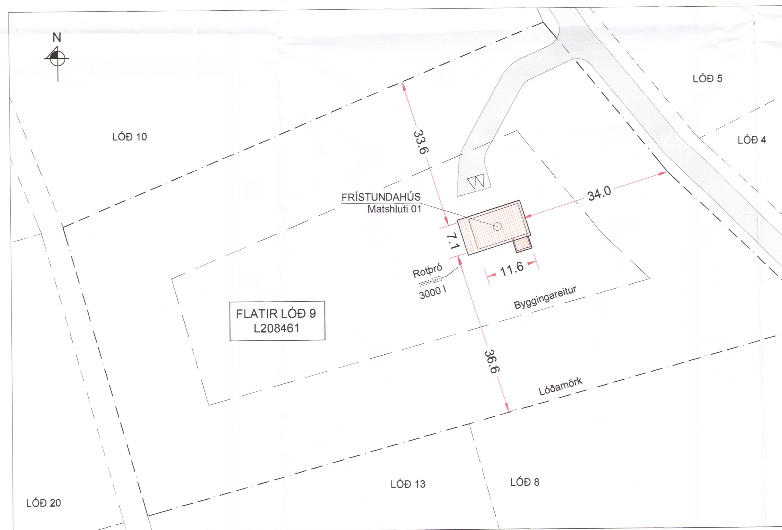
AFSTÖÐUMYND Mkv. 1:500
