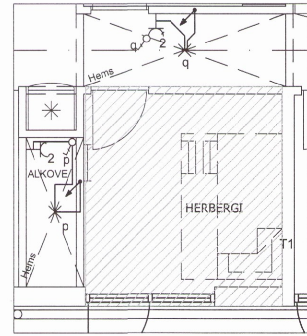
SVEFNLOFT 1:50
