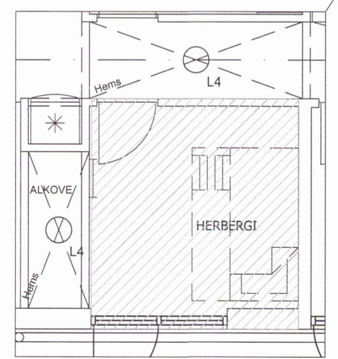
SVEFNLOFT 1:50
