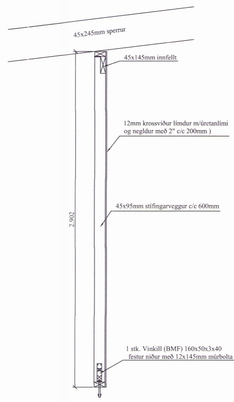
Snið í stífingurvegg mkv. 1:20
