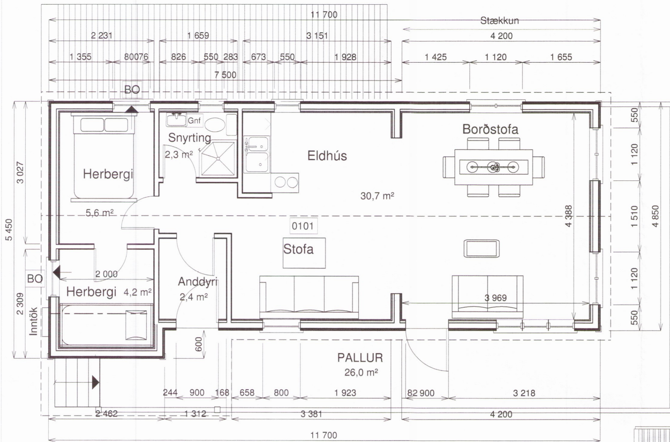
GRUNNMYND 1:50
