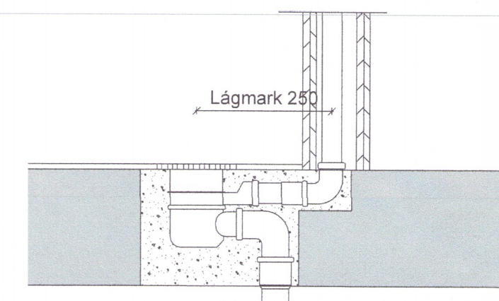
GÓLFNIDURFALL MEÐ GEGNURENSSLI, MKV.:1:10
