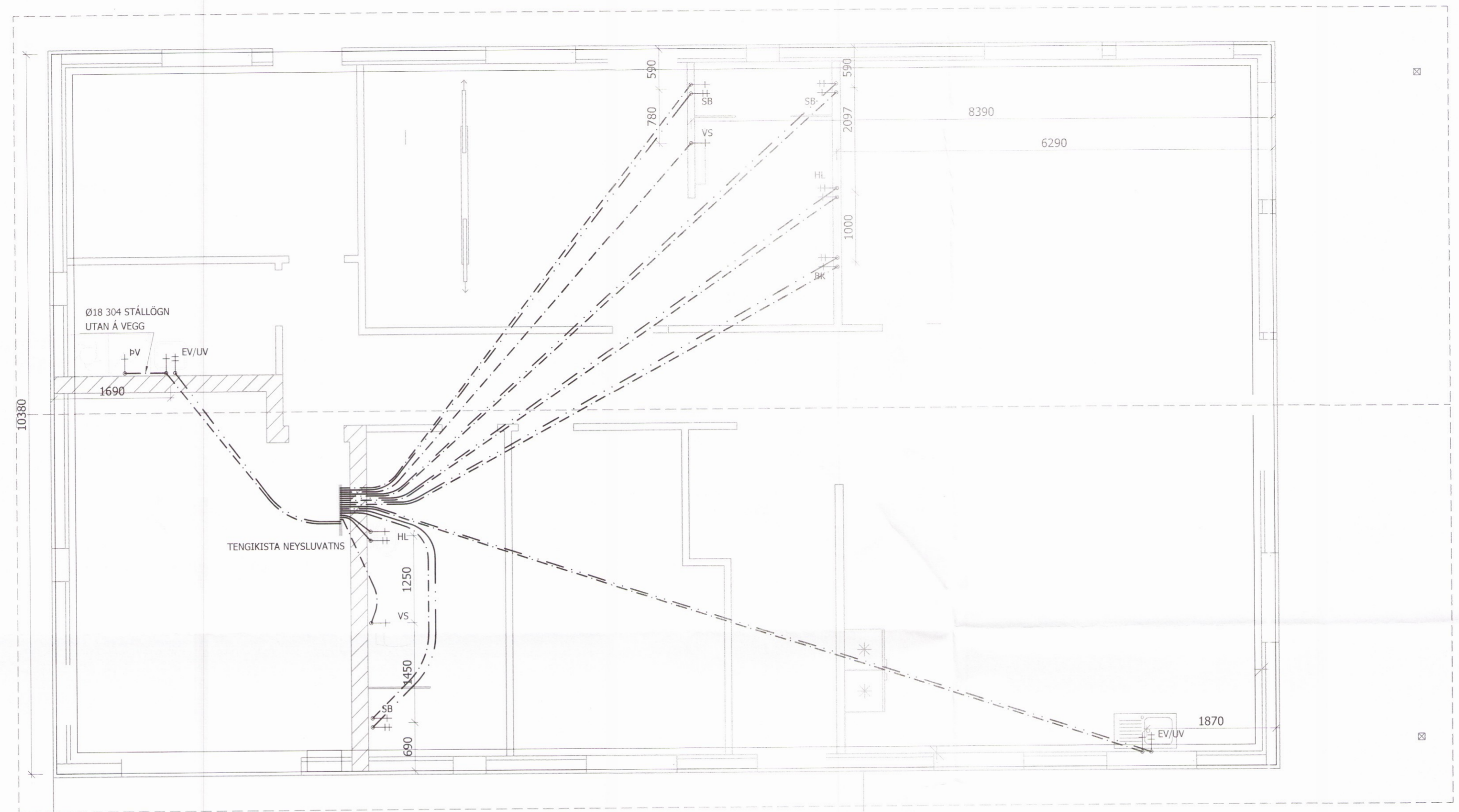
GRUNNMYND NEYSLUVATNSLAGNA
