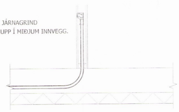
STAÐSETNING LAGNA Í PLÖTU/INNVEGG Mkv. 1:20
